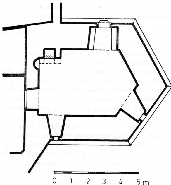
21 Tlocrt II kata peterokutne kule
