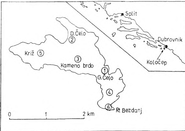
Sl. 1. Nalazišta biljnih vrsta na otoku Koločepu Fig. 1. Localities of the species on the island of Koločep
