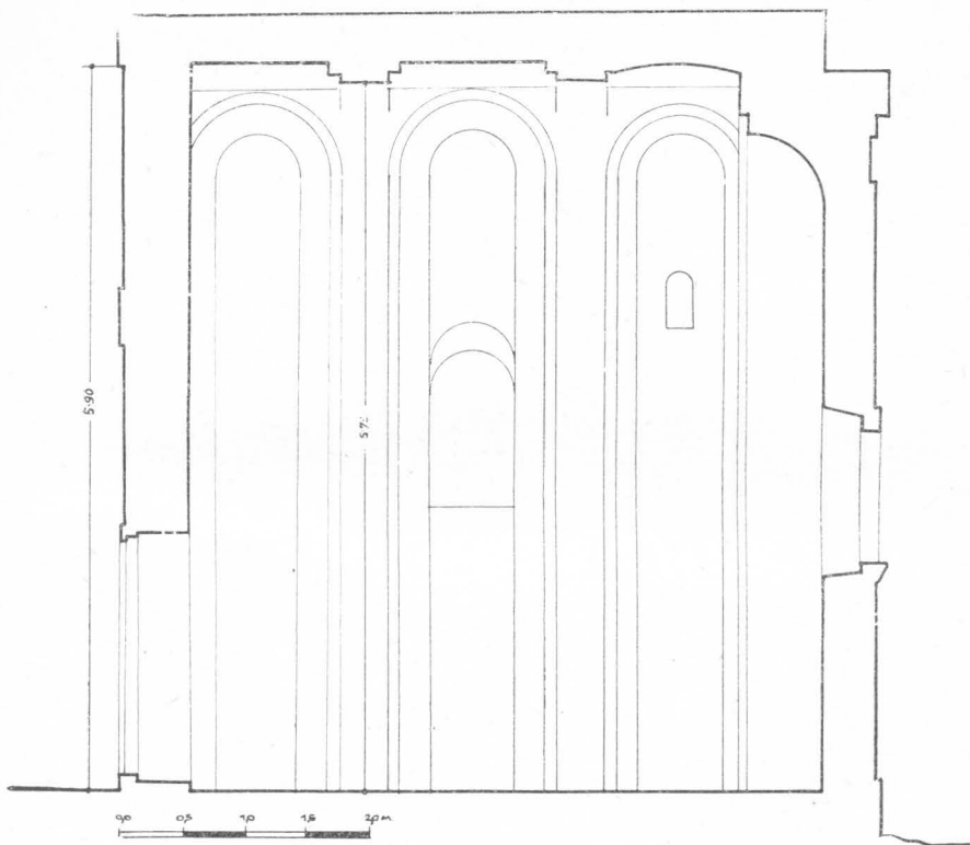
Uzdužni presjek crkvice sv. Mihajla u Stonu
