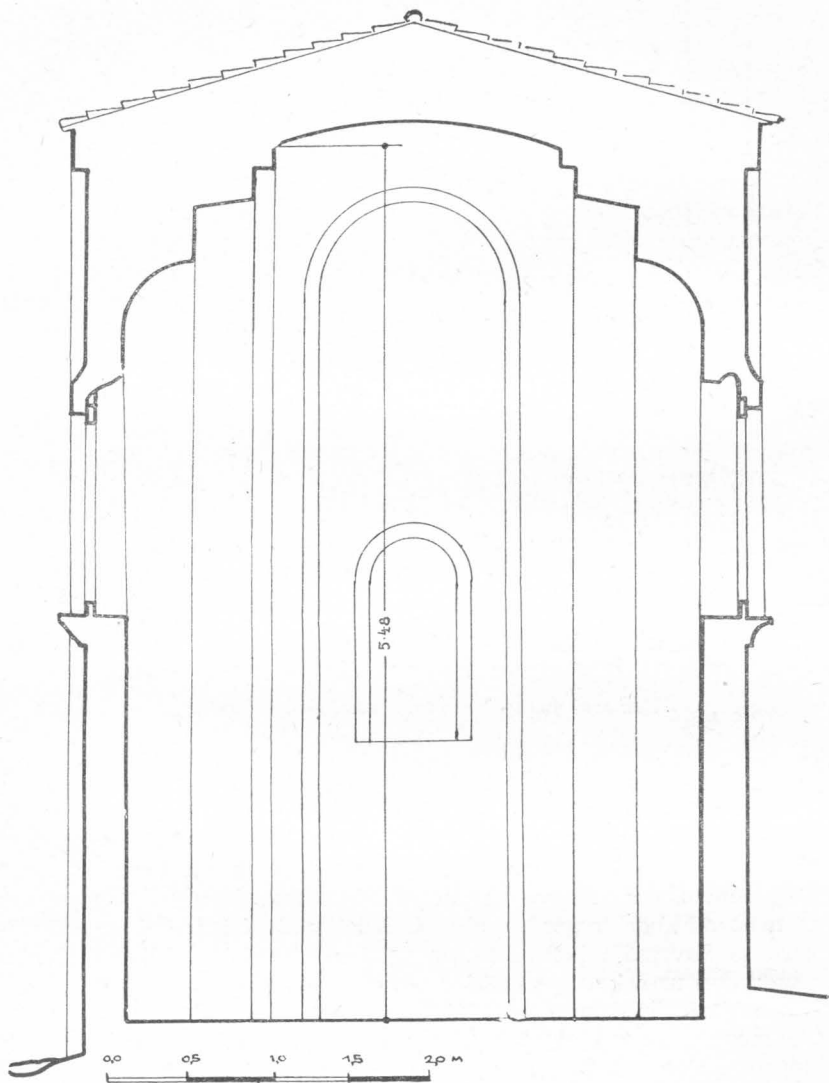
Poprečni presjek crkvice sv. Mihajla u Stonu
