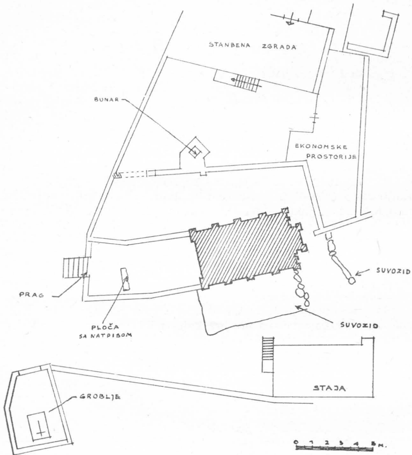
Tlocrt građevina na brežuljku sv. Mihajla u Stonu
