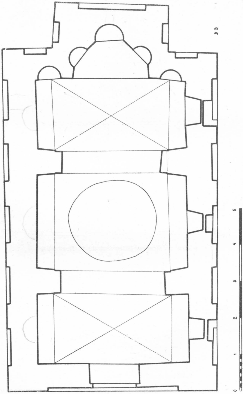
Tlocrt crkve sv. Petra na Priku u Omišu (snimio D. Domančić)
