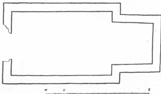
Tlocrt »Crkvine« u Lukoranu na Ugljanu
