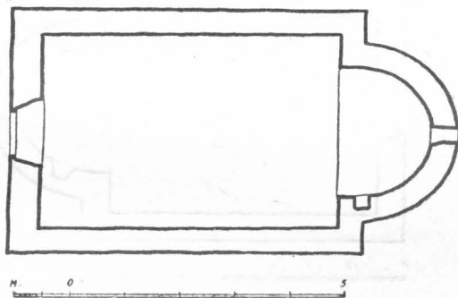
Tlocrt crkve sv. Jerolima kod Kukljice na Ugljanu
