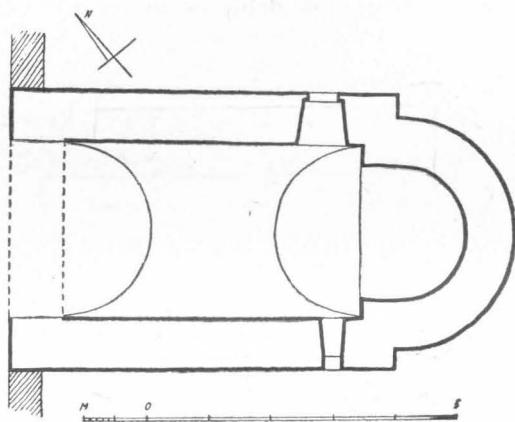
Tlocrt crkve sv. Kuzme i Damjana na Ugljanu
