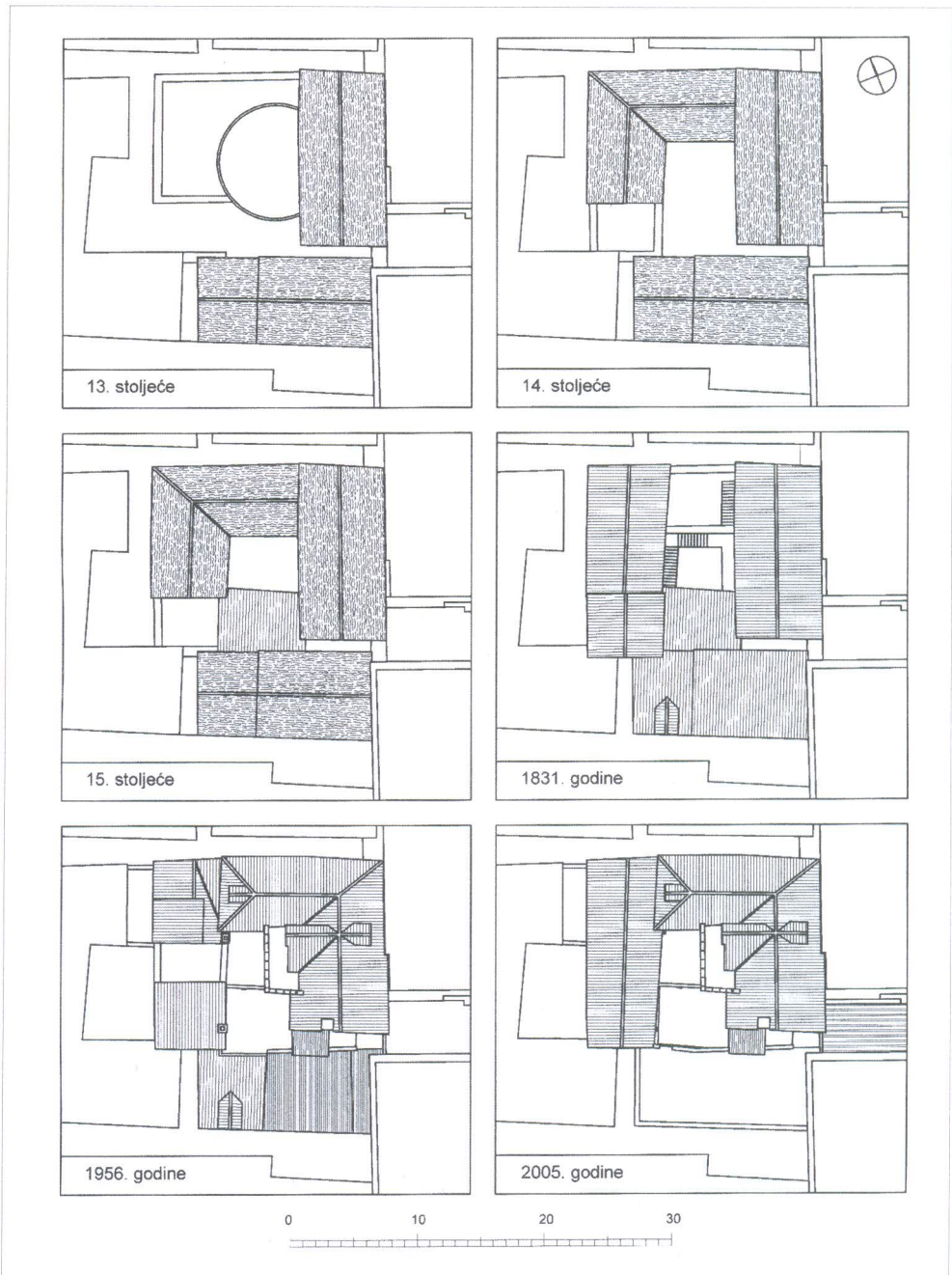
Prostorni razvoj sklopa jugozapadno od Peristila, tlocrt (K. Marasović, V. Marčić)
