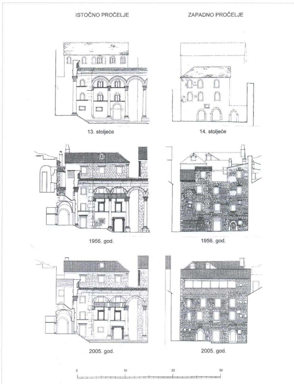
Prostorni razvoj sklopa jugozapadno od Peristila, istočno i zapadno pročelje (J. Marasović, M. Marasović, K. Marasović, V. Marčić)
