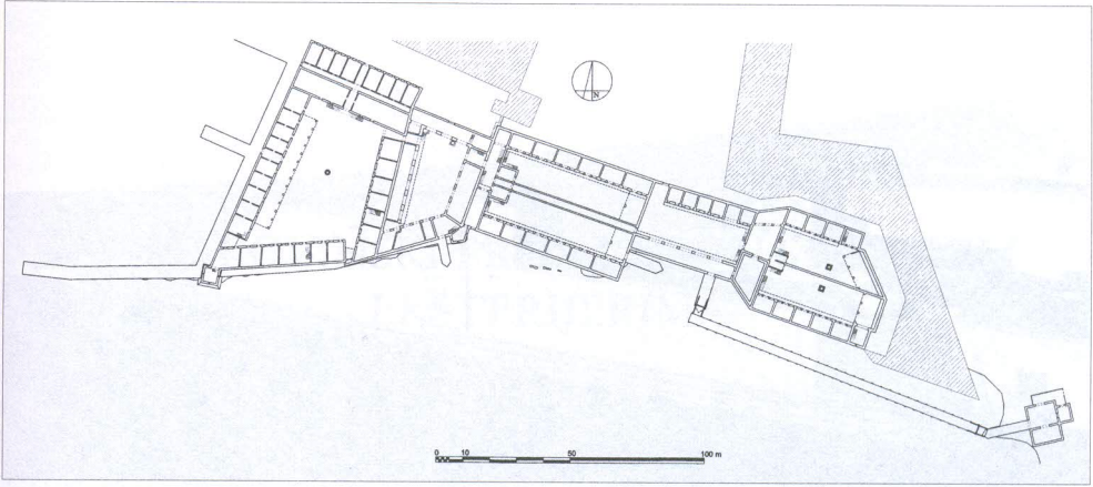
Tlocrt prizemlja lazareta, stanje 1682. godine, autor: S. Perojević, 2001.
