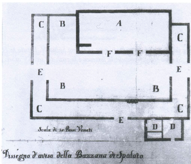
Tlocrt splitske bazane, D. Kečkemet: Zaštita od epidemija u Splitu
