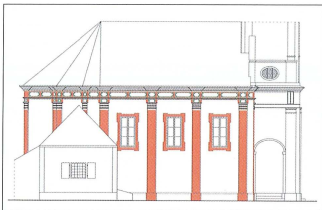
Sl. 11. Prijedlog prezentacije: zapadno pročelje
