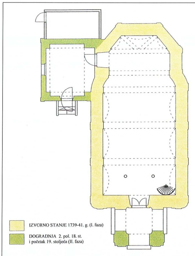
Sl. 9. Građevinske faze kapele
