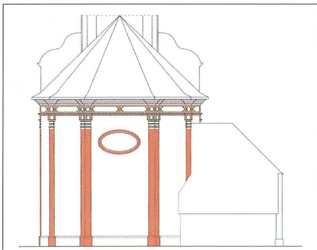
Sl. 11. Prijedlog presentacije: sjeverno pročelje
