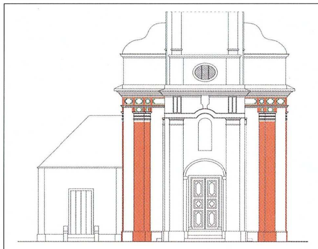
Sl. 11. Prijedlog presentacije: južno pročelje
