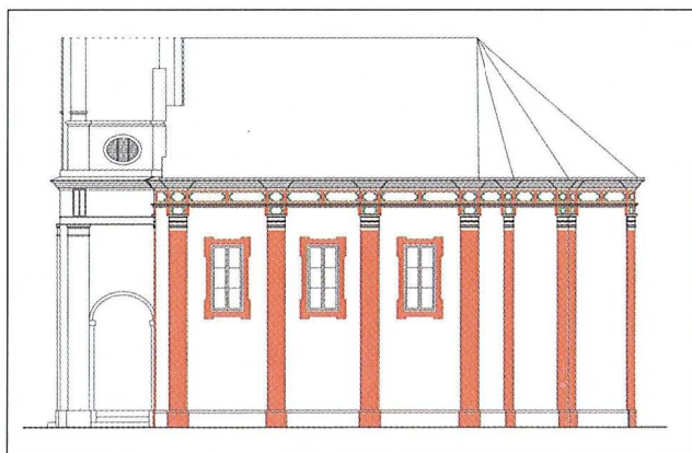
Sl. 11. Prijedlog presentacije: istočno pročelje
