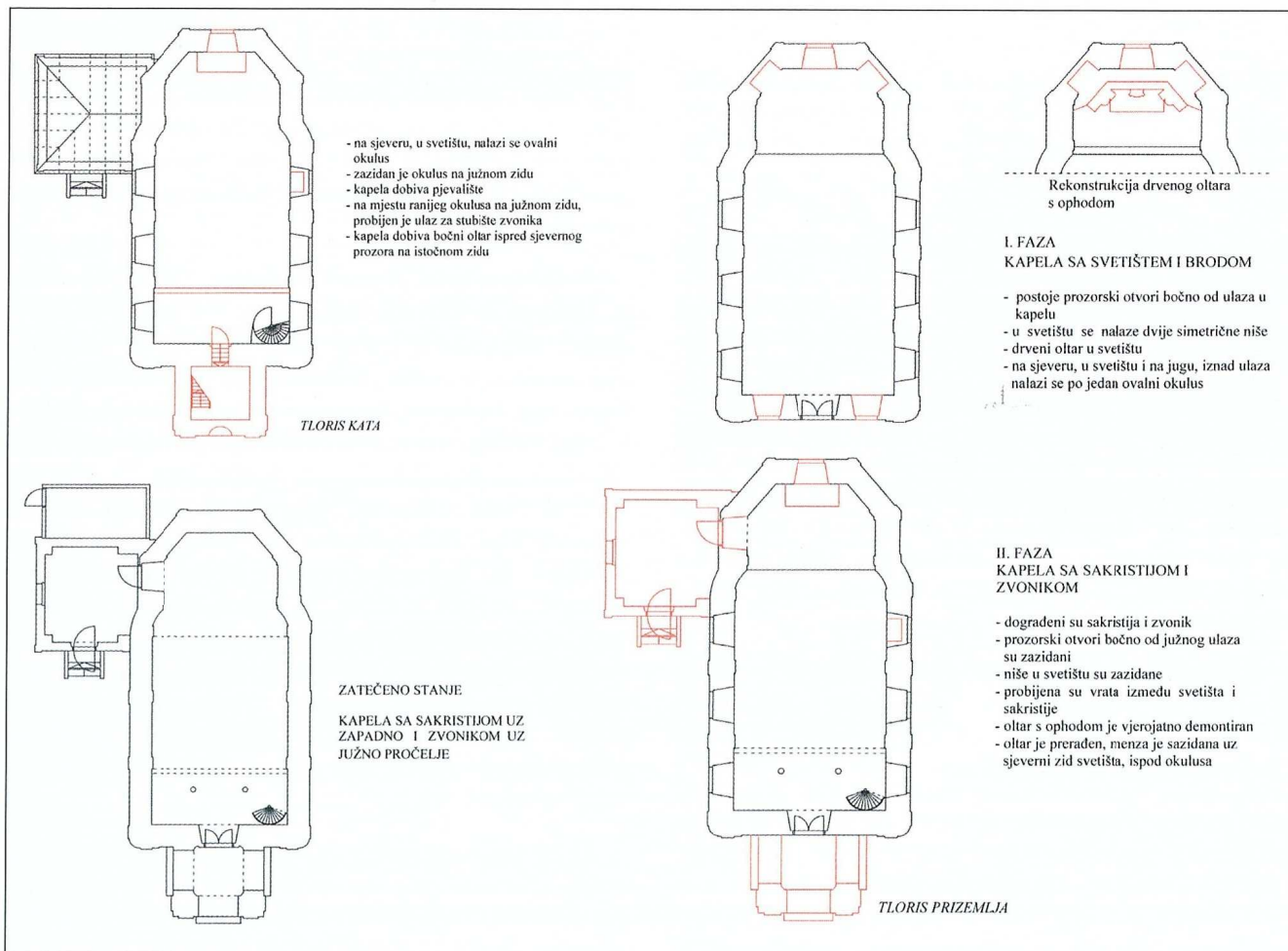
Sl. 10. Kronologija gradnje kapele
