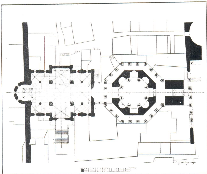
Prva varijanta Hauserovog projekta nove stolne crkve — tlocrt, foto: Ž. Bačić
