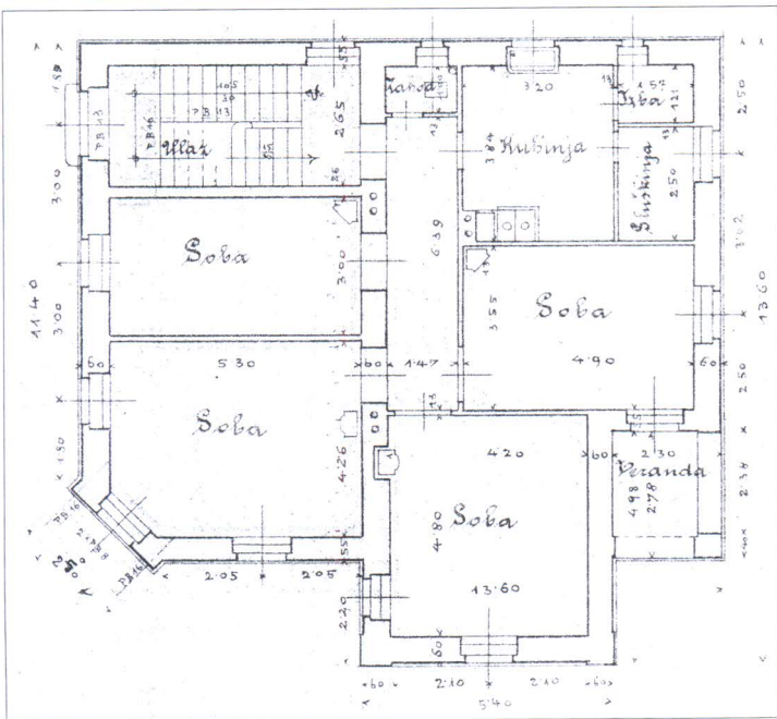
Vila M. Mikačića u Splitu na Sukoišanu. Projekt E. Žagara iz 1905. ; Južno pročelje i tlocrt prizemlja
