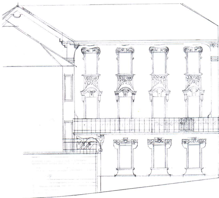
Stambena kuća Regine Arbanasović u Splitu u Čulića dvorima. Crtež južnog pročelja kojeg je napravio E. Žagar 1905. godine
