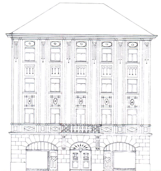
Stambena zgrada E. Karamana u Splitu. Crtež glavnog pročelja, E. Žagar 1912. godine
