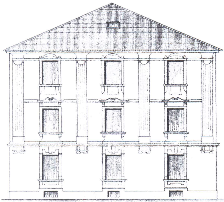
Stambena kuća braće Ferić u Splitu na Bačvicama. Nacrt E. Žagara iz 1906. godine, glavno pročelje
