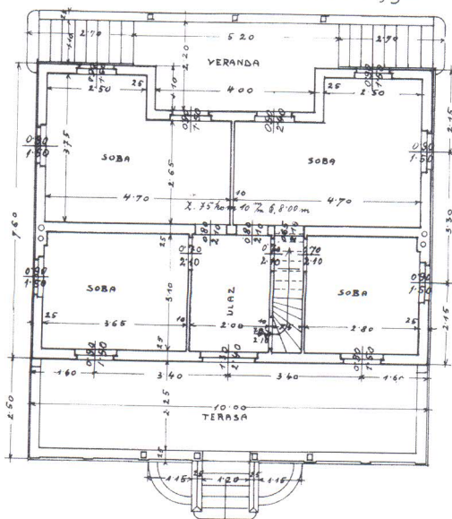
Vila I. Antičevića u Splitu na Mejama. Projekt E. Žagara 1917. godine, južno pročelje i tlocrt prizemlja
