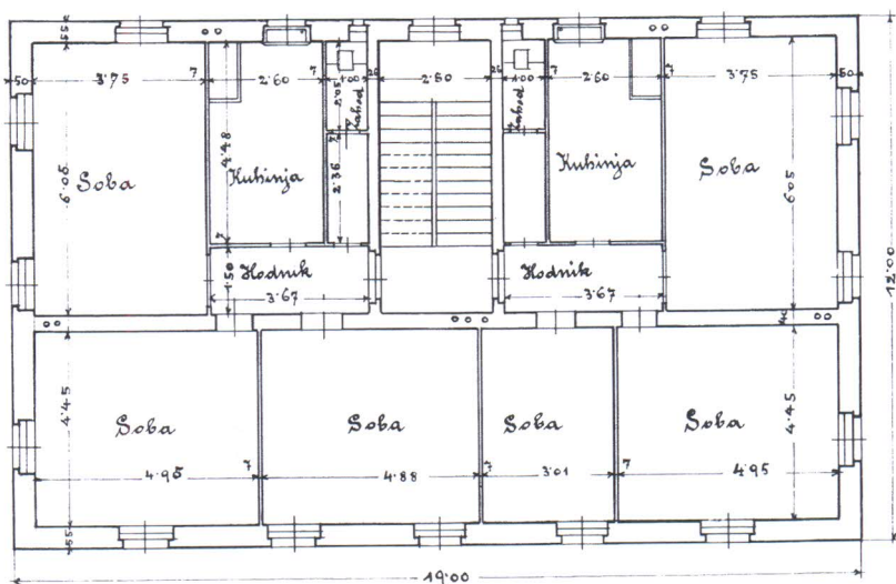
Kuća I. Dvornika uz cestu Split-Omiš. Projekt E. Žagara iz 1907. godine, tlocrt prvog kata i južno pročelje
