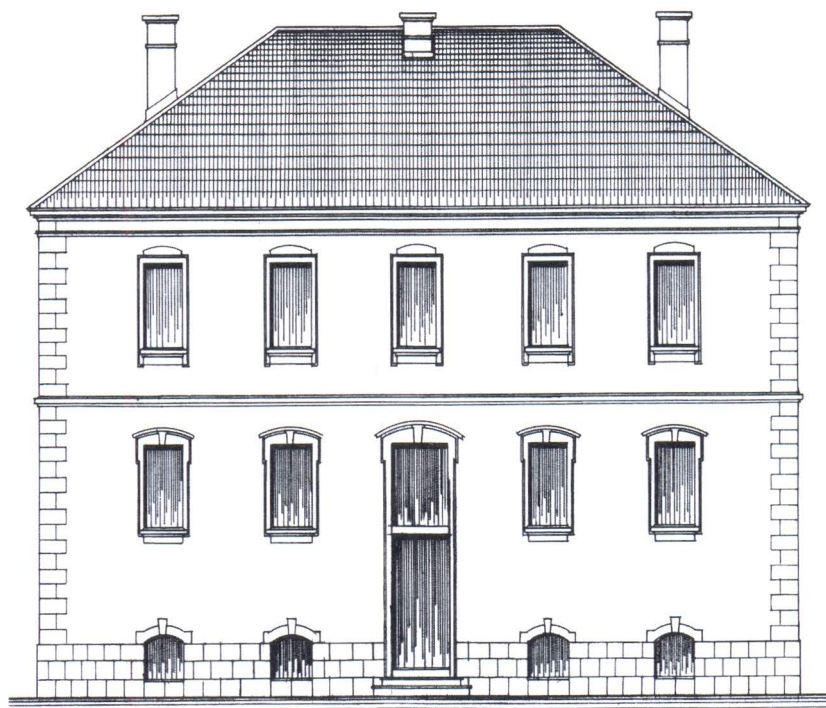
Kuća I. Dvornika uz cestu Split-Omiš. Projekt E. Žagara iz 1907. godine, tlocrt prvog kata i južno pročelje
