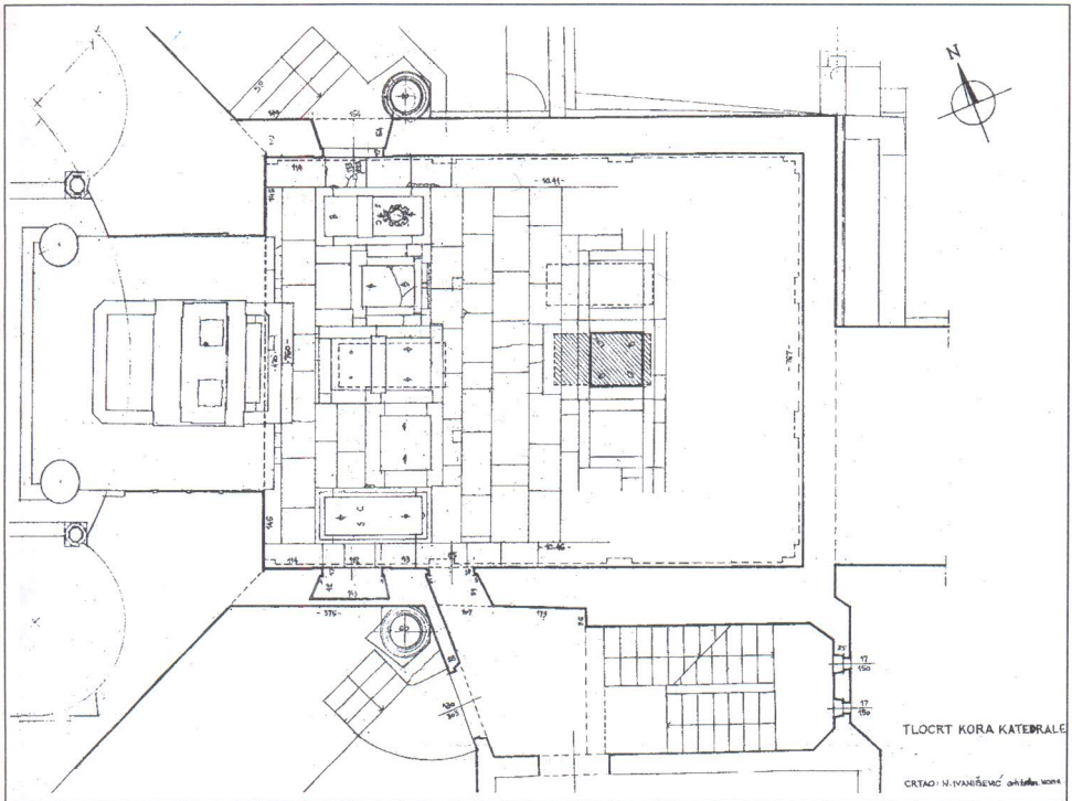
Tlocrt kora katedrale
