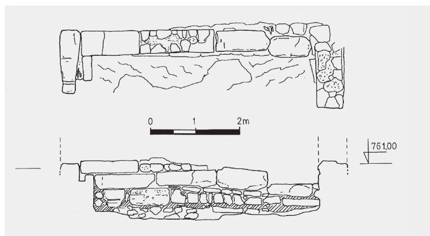
sl. 10. Uzdužni presjek i tlocrt sjevernog perimetralnog zida.
