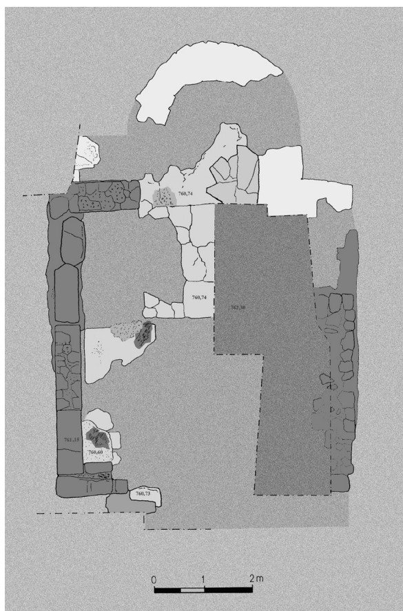
sl. 13. Tlocrt naosa nakon zahvata na arhitekturi predromaničke crkve s ostacima podnice 2a.
