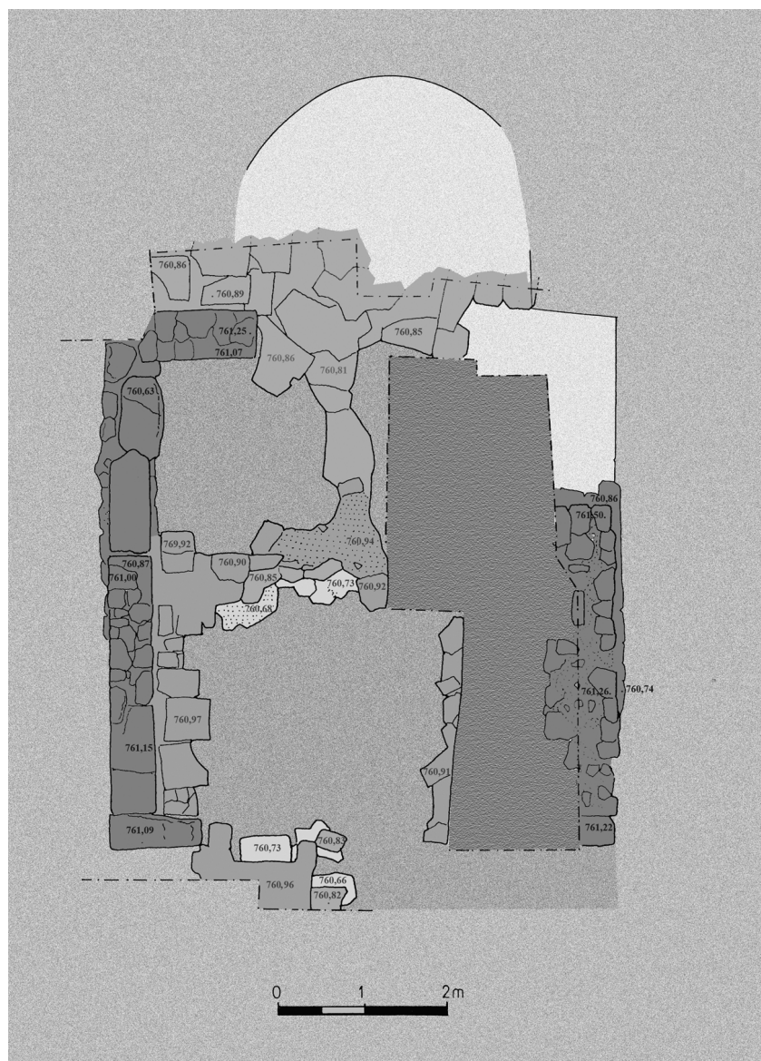
sl. 16. Tlocrt s ostacima podnica 1 i 2.
