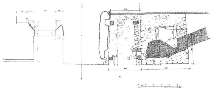
Tlocrt otkrivenih antičkih gradskih vrata u Ninu
