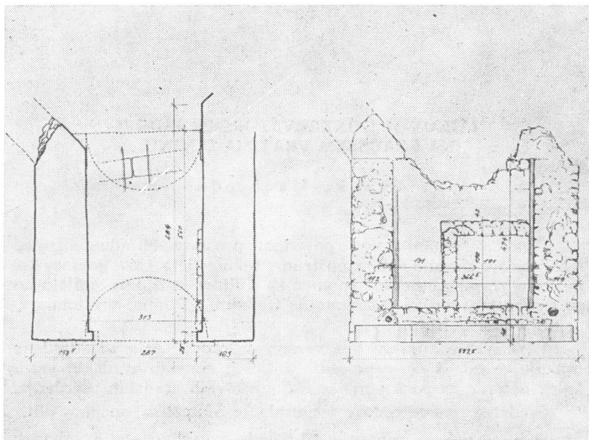
Nin, Donja vrata, tlocrt prizemlja i prvog kata kule
