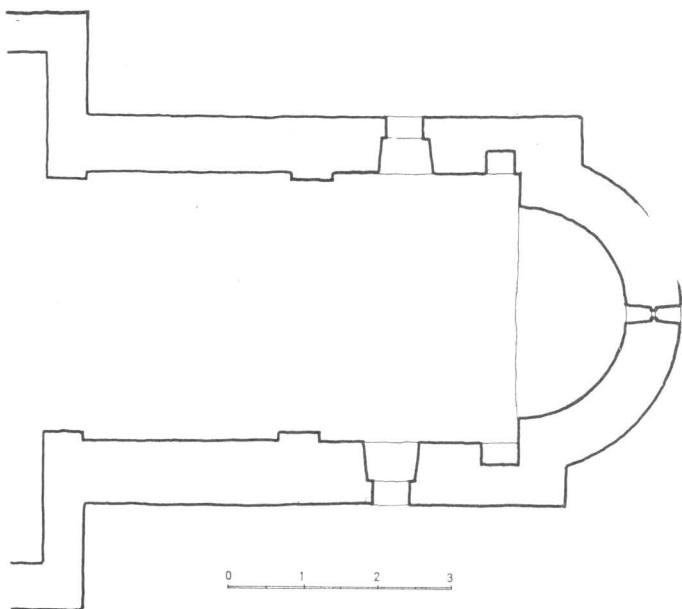
Crkvice Sv. Jure u Prhovu, tloris
