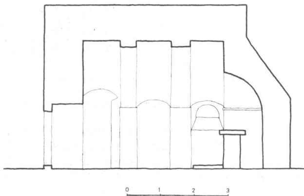
Tlocrt i uzdužni presjek crkvice Sv. Ivana na rtu Planke
