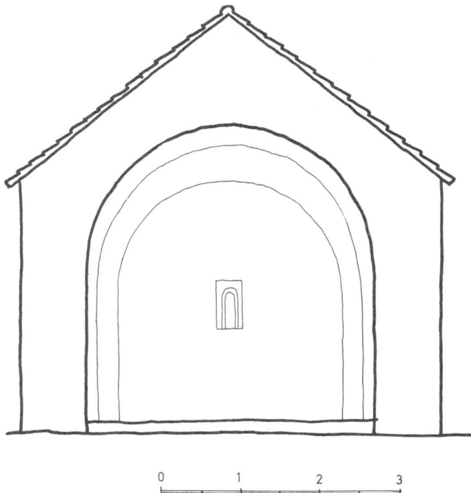
Crkvice Sv. Jure u Prhovu, poprečni presjek
