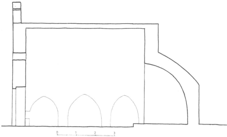
Crkvice Sv. Nikole u Rogoznici, uzdužni presjek
