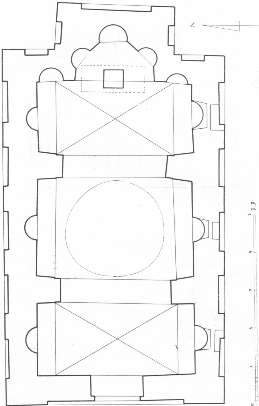
Omiš, Tloris crkve sv. Petra na Priku (snímio D. Domančić)
