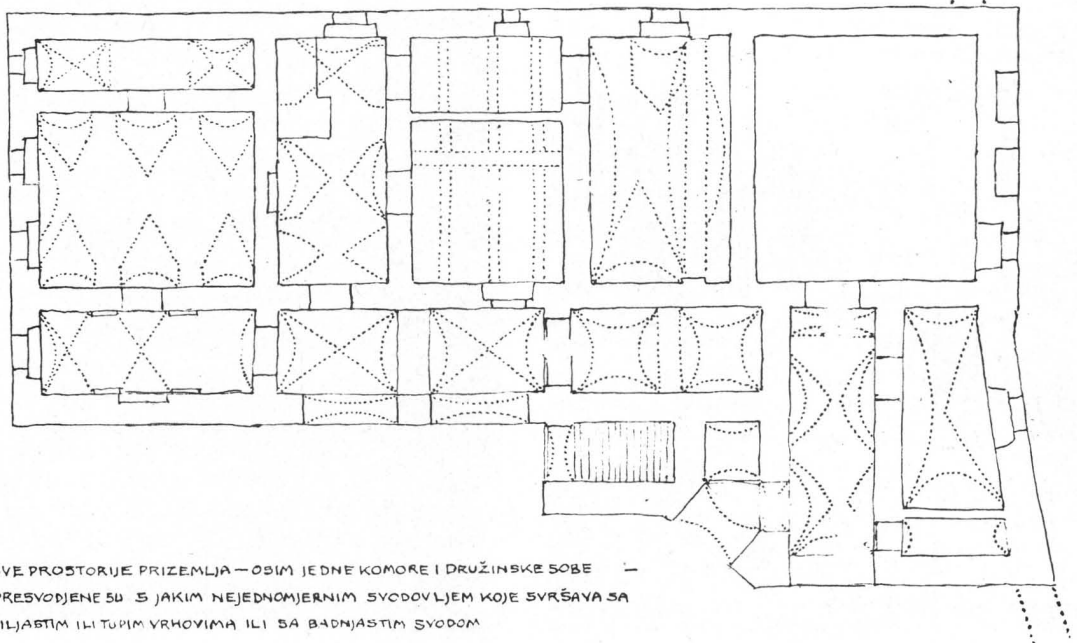
Kaptol 22, tlocrt prizemlja
