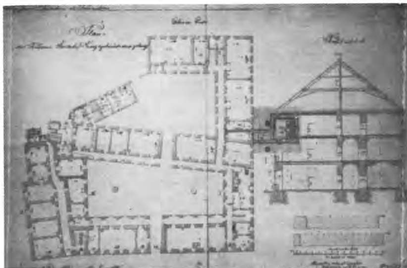
11 Petrovaradin, tlocrt prizemlja bivšeg franjevačkog samostana s dogradnjama 1874. godine — Ratni arhiv u Beču
