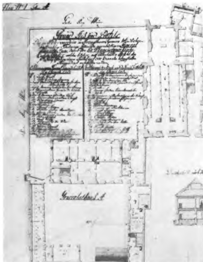
6 Petrovaradin, tlocrt franjevačke crkve preuređene za žitnicu, kraj XVIII. st. — Ratni arhiv u Beču
