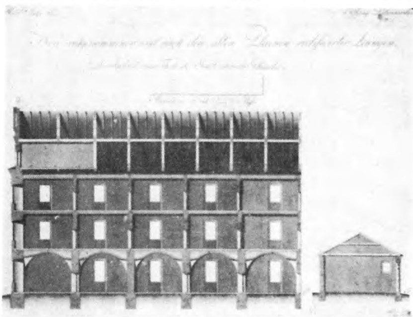
9 Petrovaradin, crkva sv. Franje nakon pregradnje, uzdužni presjek 1820. godine — Ratni arhiv u Beču
