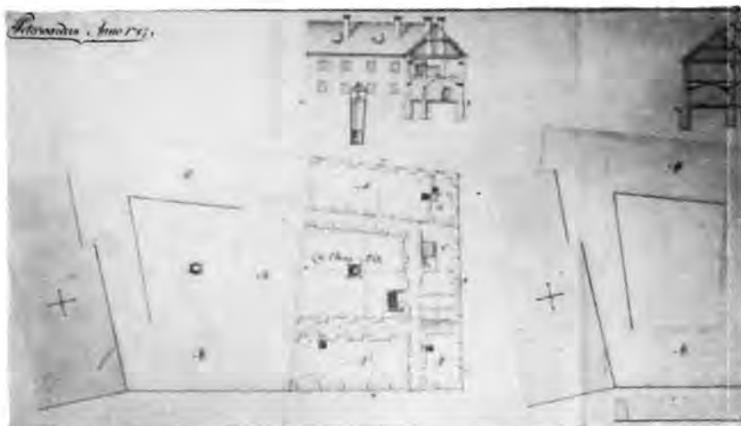
4 Petrovaradin, prizemlje oduzetog i dograđenog novog dijela franjevačkog samostana za vojnu bolnicu. Izgled sjevernog krila i poprečni presjek južnog krila 1783/84. godine
