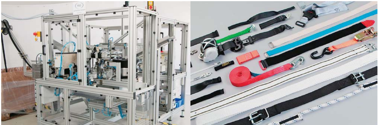
Sl.1 Proizvodna linija "Narrow-Matic" tvrtke RSG za automatsko prerađivanje i konfekcioniranje proizvoda - traka za podizanje tereta i vezanje, sigurnosni pojasevi, gurta za penjanje i medicinskih tekstilija
