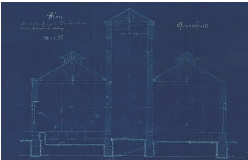
Slika 7. Strojarnica za hidrauličko postrojenje, 1884., poprečni presjek [11]
