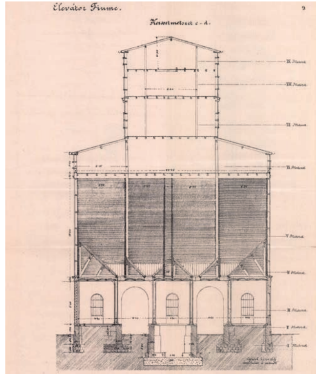
Slika 16. Žitni silos, poprečni presjeci c-d [16]
