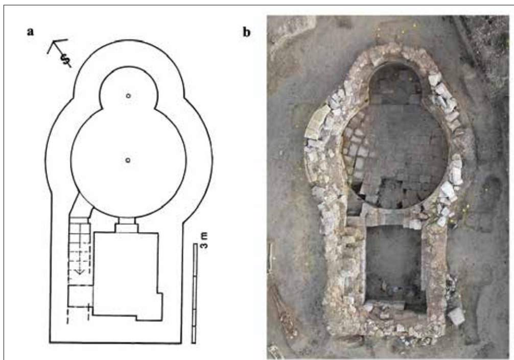
4 Tlocrt rotunde na lokalitetu „Njive“ - Ivaldola: a) donja etaža, arhitektonska snimka (zanemarena su oštećenja, crtež: Z. Horvat); b) zračna snimka rotunde (foto: M. Hucaljuk)
