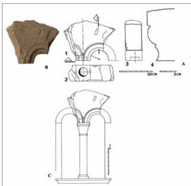
11 Ulomak bifore (?), pronađen na lokalitetu „Njive“ - Ivandol: A) arhitektonska snimka: 1-pogled sprijeda, 2-pogled odozdo, 3-presjek, 4-detalj profilacije; C) pokušaj rekonstrukcije bifore (crtež: Z. Horvat); B) fotografija ulomka (foto: M. Mihaljević)
