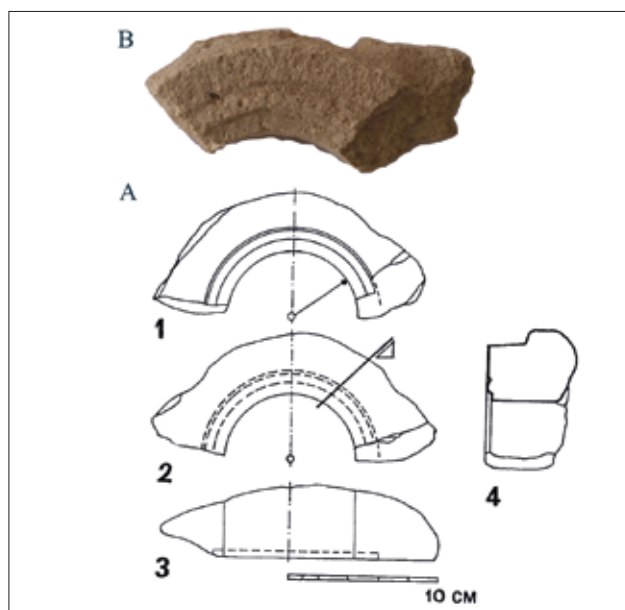
13 Ulomak malog luka (možda svetohraništa ili zidne niše), pronađen na lokalitetu „Njive“ - Ivandol: A) arhitektonska snimka: 1-pogled sprijeda, 2-pogled straga, 3-pogled odozdo, 4-presjek (crtež: Z. Horvat); B) fotografija ulomka (foto: M. Mihaljević)
