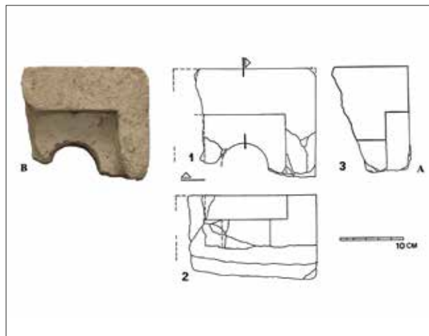
12 Ulomak tranzene prozora (?), pronađen na lokalitetu „Njive“ - Ivandol: A) arhitektonska snimka: 1-pogled sprijeda, 2-pogled odozdo, 3-presjek (crtež: Z. Horvat); B) fotografija ulomka (foto: M. Mihaljević)
