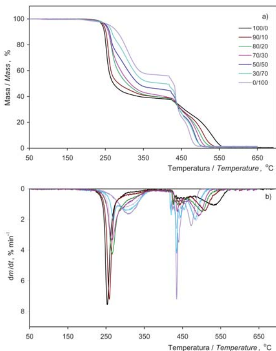
SLIKA 3. Dinamičke TG (a) i DTG (b) krivulje termooksidacijske razgradnje mješavina PVC/CPE bez stabilizatora; brzina zagrijavanja 2,5 \text{ }^\circ\text{C min}^{-1} FIGURE 3. Dynamic TG (a) and DTG (b) curves for thermooxidative degradation of PVC/CPE blends without stabilizer; heating rate 2,5 \text{ }^\circ\text{C min}^{-1}
