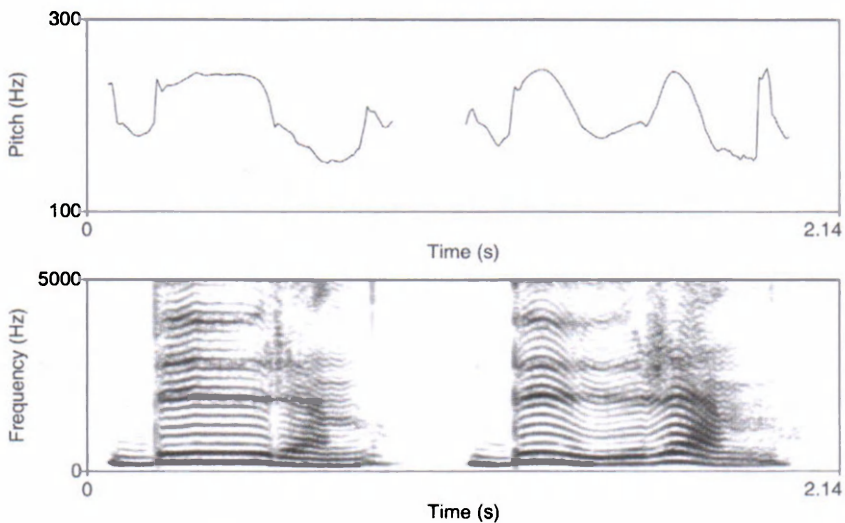
Slika 4b. Akustički prikaz švedskih naglasaka: 'buren (akcent 1) 'krletke', `buren (akcent 2) 'nošen' Figure 4b. Acoustics of Swedish accents: 'buren (accent 1) 'cages', `buren (accent 2) 'carried'
