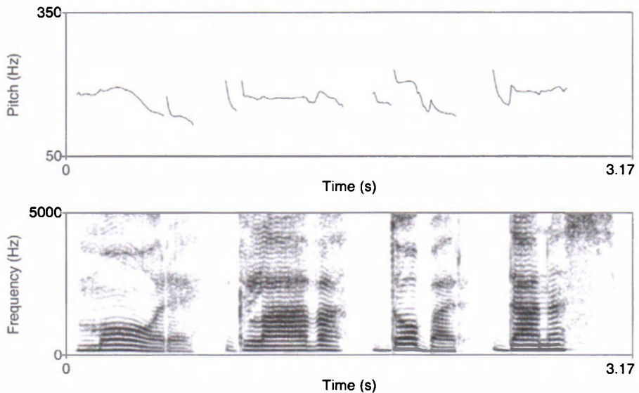
Slika 1b. Akustički prikaz hrvatskih naglasaka: mōre (ds), glāva (du), dōbar (ks), danas (ku)
