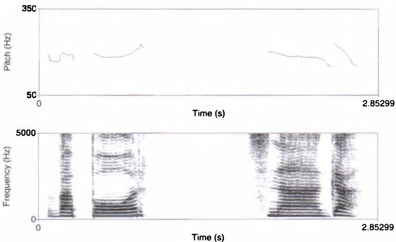
Slika 6c. Akustički prikaz hrvatskih čakavskih naglasaka (na zadnjem slogu u riječi): vapōr (akut), snāgā (ks)
