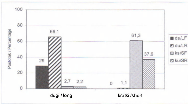
Slika 2c. Percepcija čeških dugih i kratkih naglašenih vokala Figure 2c. Perception of Czech long and short stressed vowels
