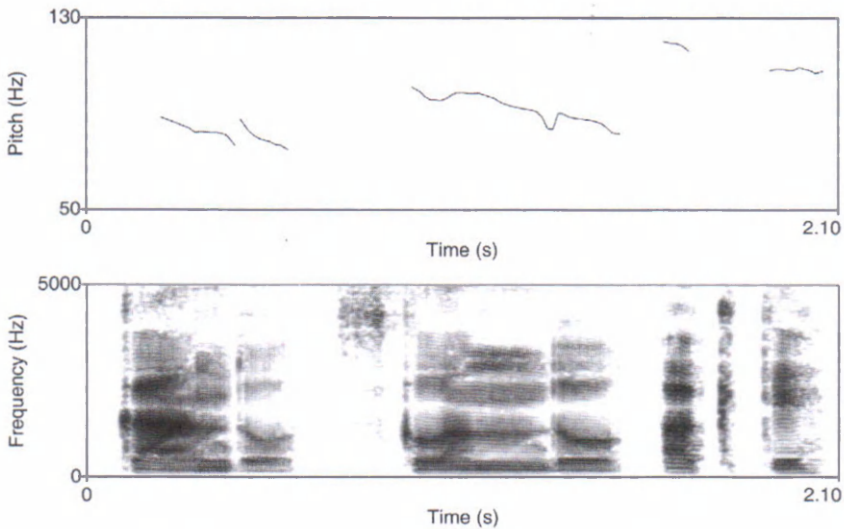
Slika 3b. Akustički prikaz litavskih naglasaka: kándo (akut) 'grizao je', sklándo (cirkumfleks) 'on lebdi', ákti (gravis) 'slijepiti' Figure 3b. Acoustics of Lithuanian accents: kándo (acute) 'he bit', sklándo (circumflex) 'he flies', ákti (grave) 'to become blind'
