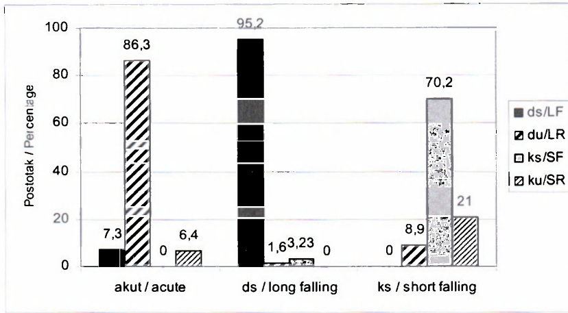
Slika 6a. Percepcija hrvatskih čakavskih naglasaka (iz Vele Luke) Figure 6a. Perception of Croatian Čakavian accents (from Vela Luka)
