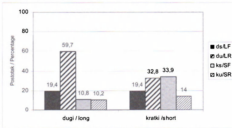
Slika 2a. Percepcija engleskih dugih i kratkih naglašenih vokala Figure 2a. Perception of English long and short stressed vowels
