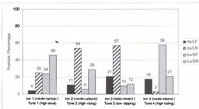
Slika 7a. Percepcija četiriju kineskih tonema (pekinški, mandarinski kineski) Figure 7a. Perception of four Chinese tones (Peking Mandarin Dialect)
