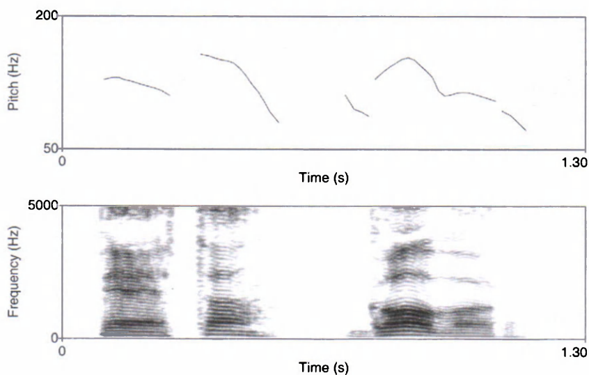
Slika 5b. Akustički prikaz slovenskih naglasaka: péta (akut), gôvor (cirkumfleks)
