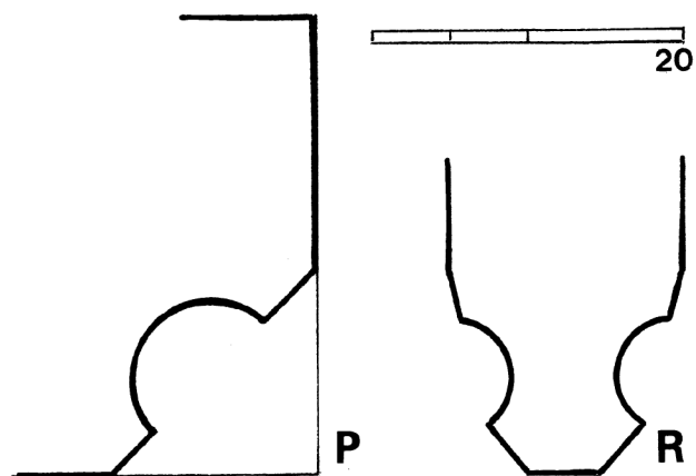
Sl. 15 Profilacije pojedinih kamenih detalja Sv. Ivana: P - profilacija zapadnog portala; R - profilacija rebra svoda, nađena u nasipu svetišta prigodom radova 1995. godine (crtež: Z. Horvat prema snimku Z. Baloga iz 1995. g.)
