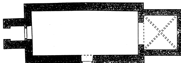
Sl. 21 Prijedlog Z. Baloga o mogućem izgledu tlocrta svetišta crkve Sv. Ivana: prema zakrivljenosti elementa rebra zaključuje da bi se ono moglo usporediti s više identičnih tlocrta crkava u potkalničkom kraju (crtež: Z. Balog, 2003.)
