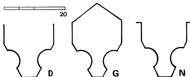
Sl. 20 Profilacije rebara, sličnih onome nađenom u podu svetišta crkve Sv. Ivana prigodom radova 1990. g.: Đ – Đurđić, spolij; G – Gornji Križ kod Zrinskog Topolovca, spolij; N – župna crkva u Novigradu na Dobri (crtež: Z. Horvat)
