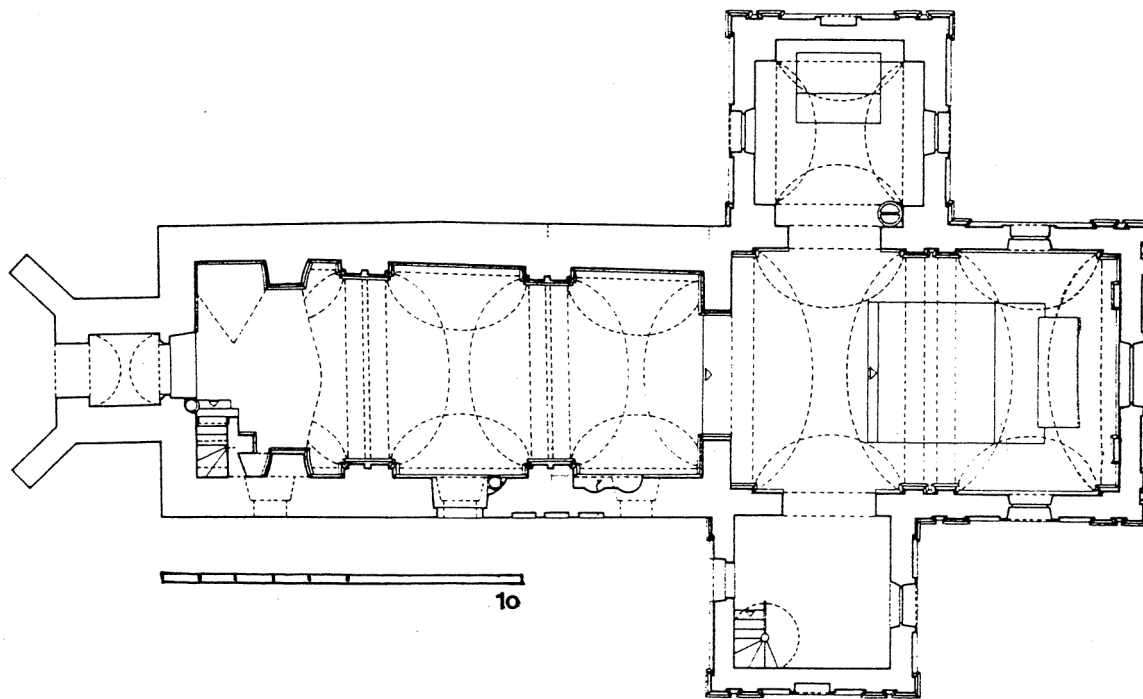
Sl. 1 Župna crkva Sv. Ivana Krstitelja u Žabnu, tlocrt (crtež: D. Stepinac, u: K. Horvat-Levaj 1993: 370) Fig. 1 St. John the Baptist Parish Church in Žabno, layout (drawing: D. Stepinac, in: K. Horvat-Levaj 1993: 370)
