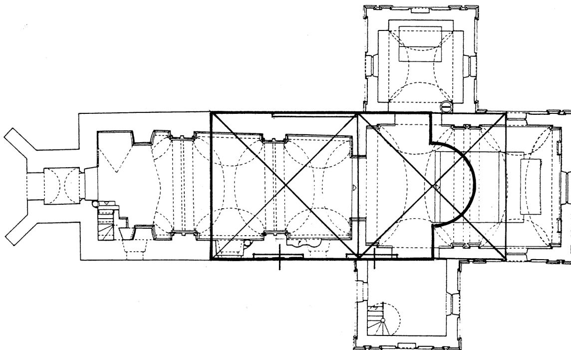
Sl. 18 Pokušaj kvadrangulacije tlocrta današnjeg stanja te tlocrta romaničko-gotičke crkve iz sredine 15. st. prema raspoloživim podacima: osnovni je kvadrat veličine 4 hvata/4 hvata, te se pojedinostima na sjevernom i južnom pročelju, slijepim nišama i dr. dobro uklapa u faze gradnje (kvadrangulacija Z. Horvata na podlozi snimka D. Stepinca)
