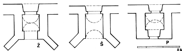
Sl. 23 Tlocrti prizemlja nekih zvonika, identičnih veličina: Ž – Sv. Ivan Žabno; Š – Novo Štefanje, župna crkva Sv. Stjepana; P – Perušić, župna crkva Sv. Križa Fig. 23 Ground plan of some belfries of identical sizes: Ž – Sv. Ivan Žabno; Š – Novo Štefanje, St. Stephen's Parish Church; P – Perušić, St. Cross Parish Church
