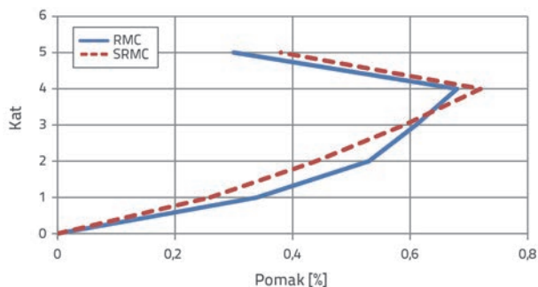
Slika 5. Usporedba međukatnih pomaka za okvir s ekscentričnim vezom u obliku obrnutog slova V
