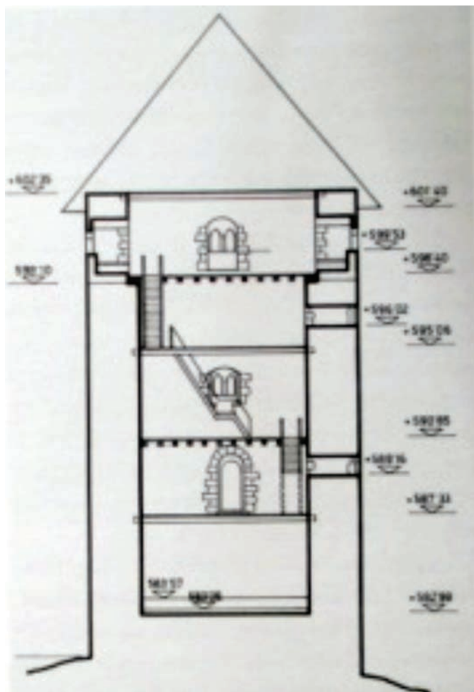
Južna kula: presjek s pogledom prema sjeveru prema Mariji Valjata Fabris
