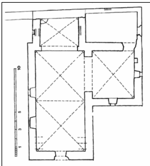
Sl. 2. Tloris crkve sv. Filipa i Jakova (prema Z. HORVAT, 2001.)
