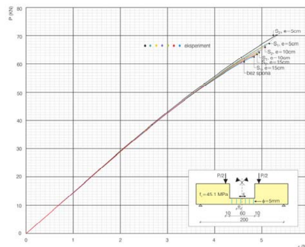
Slika 13. Izmjerene vrijednosti veze sila ( P ) – tlačna deformacija betona ( \epsilon ) kod greda od betona f_c = 45,1 MPa
