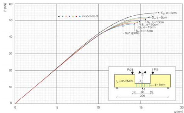
Slika 9. Izmjerene vrijednosti veze sila ( P ) – pomak ( \Delta ) kod greda od betona f_c = 35,2 MPa
