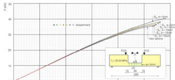
Slika 11. Izmjerene vrijednosti veze sila ( P ) – tlačna deformacija betona ( \epsilon ) kod greda od betona f_c = 24,9 MPa
