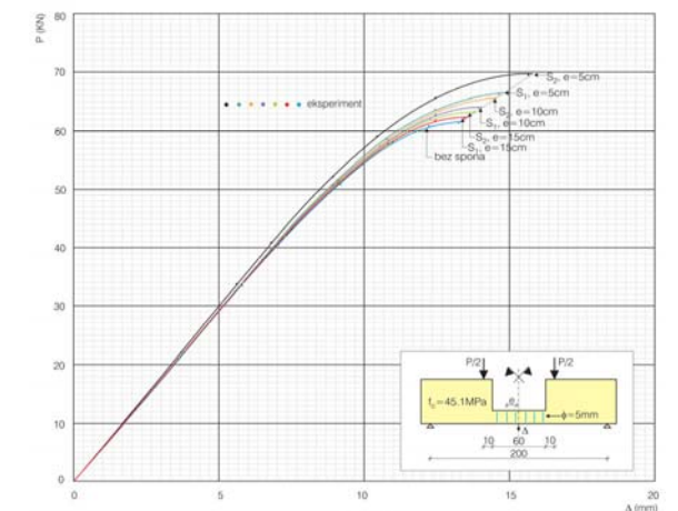
Slika 10. Izmjerene vrijednosti veze sila ( P ) – pomak ( \Delta ) kod greda od betona f_c = 45,1 MPa
