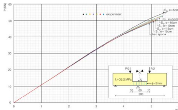
Slika 12. Izmjerene vrijednosti veze sila ( P ) – tlačna deformacija betona ( \epsilon ) kod greda od betona f_c = 35,2 MPa
