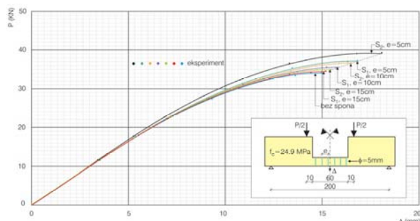
Slika 8. Izmjerene vrijednosti veze sila ( P ) – pomak ( \Delta ) kod greda od betona f_c = 24,9 MPa
