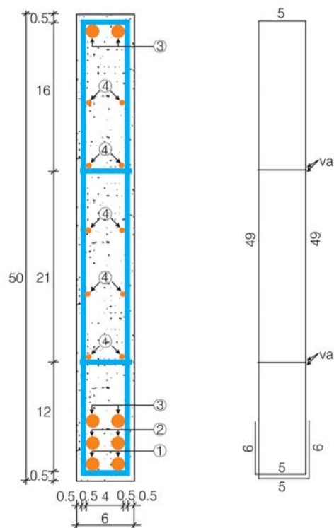
Slika 4. Poprečni presjek grede uz oslonce
