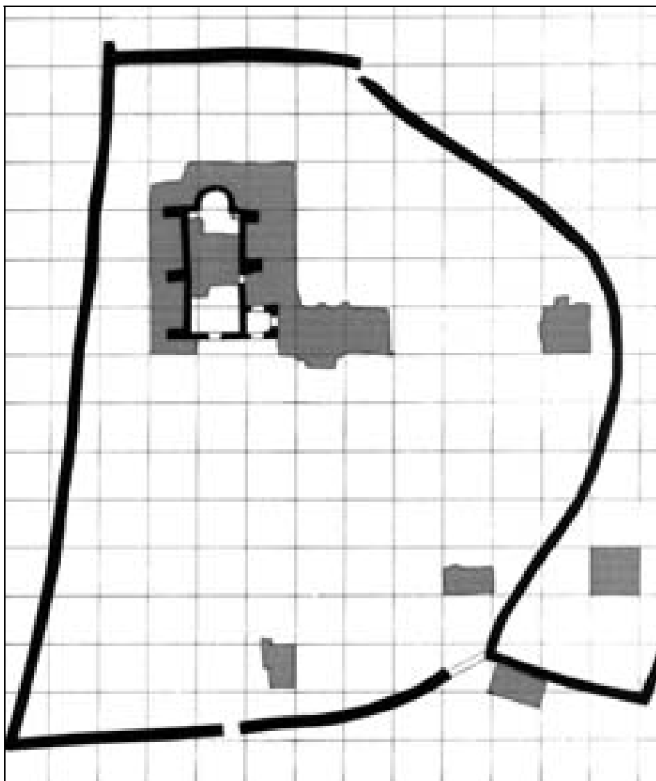
Sl. 1. Tloris crkve sv. Petra u Starigradu i istraživanih sondi godine 1999. (J. Vučić)
