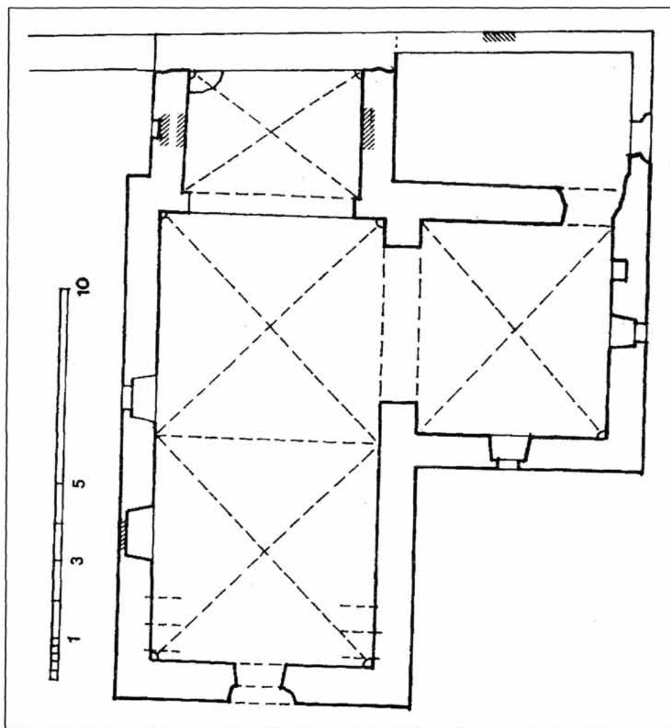
Sl. 1. Sveti Juraj, crkva sv. Filipa i Jakova, tlocrt (crtež Z. Horvat)
