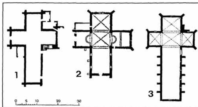
Sl. 8. Tlocrti nekih ženskih cistercijskih samostana (prema A. DIMIER, 1967.): 1. Le Savouir, Francuska, 13. st.; 2. Le Miroir, Francuska, 12. st.; 3. Cadins, Španjolska, 13. st.
