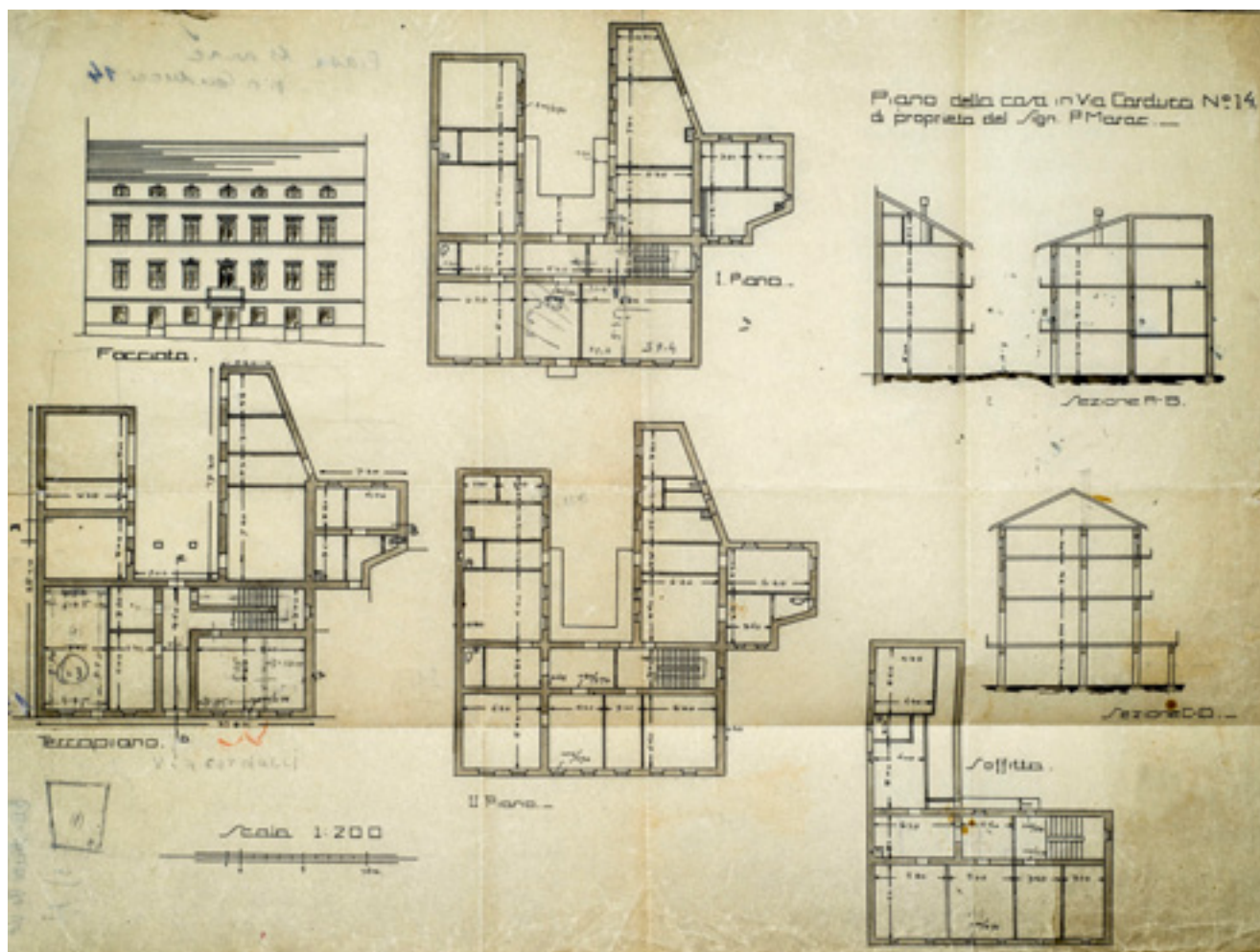
10. Nacrt bivše Gerliczyjeve palače iz 1930. kada je ona u vlasništvu Petra Marca (izvor: Državni arhiv u Rijeci)
