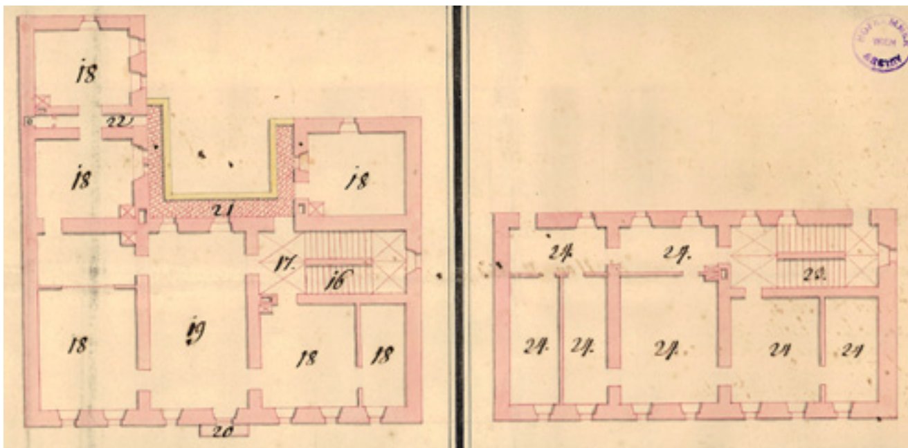
3. Tlocrti prvog i drugog kata palače Gerliczy, detalj nacrtu Plan des Baron Gerlitzyschen Haus in Fiume , 1780. (izvor: Österreichisches Staatsarchiv, Hofkammerarchiv, Beč)
