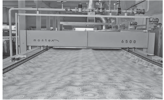
Sl.1 Nabavom rasteznog sušionika Montex 6500 Vicenta home udvostručuje proizvodnju
