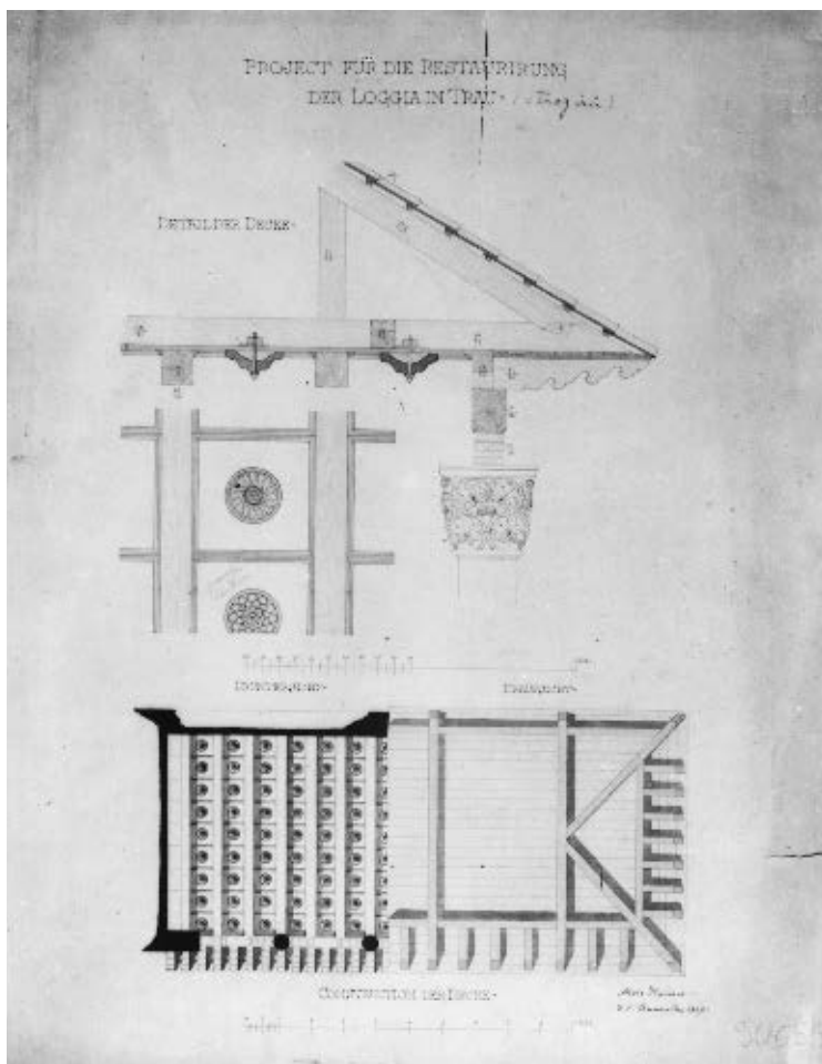
Projekt obnove gradske lože u Trogiru. (Arhiv Konzervatorskog odjela u Splitu)
