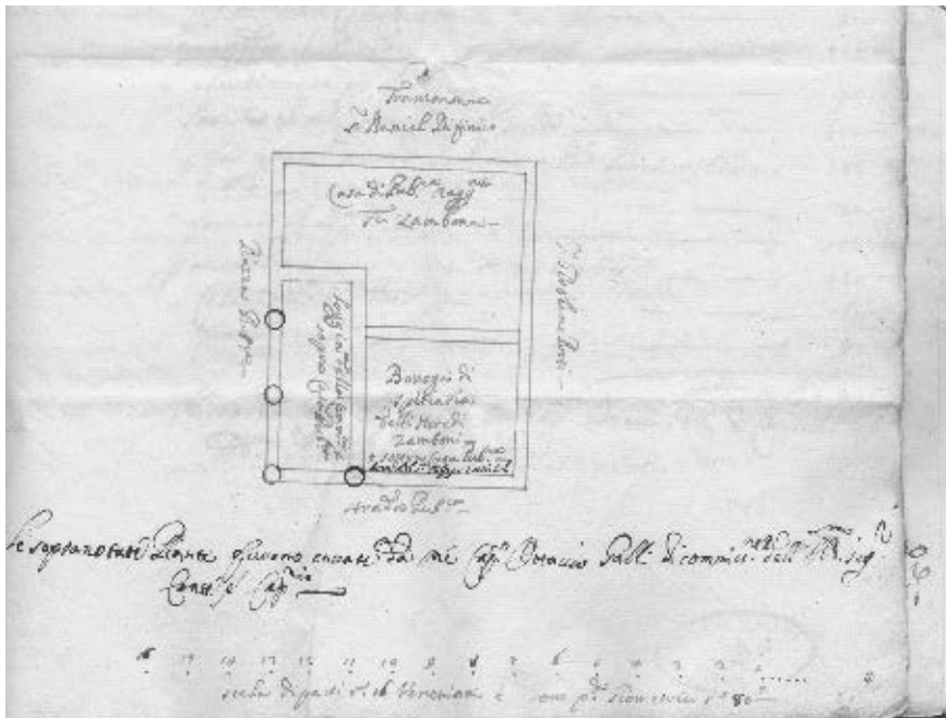
Skica šibenske male lože, XVII. st. (Archivio di Stato di Venezia)
