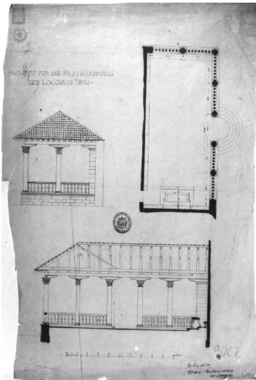
Projekt obnove gradske lože u Trogiru. A. Hauser, 1890. (Arhiv Konzervatorskog odjela u Splitu)
