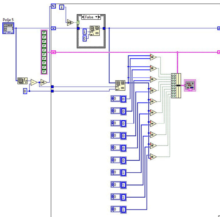
Slika 4 Dio programa korišten za prepoznavanje pritiska tipki dalj. upr.
