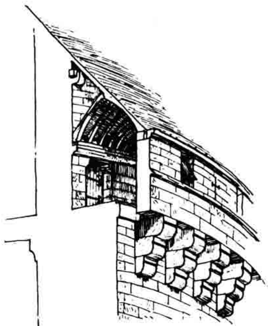
Sl. 135. — Proširenje kule na vrhu kamenim zidom na konzolama (prema Viollet le Ducu).
