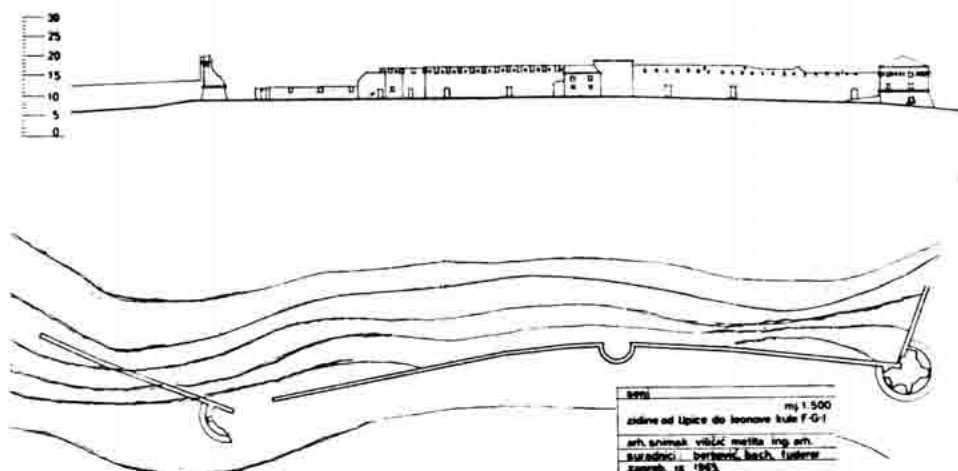
Sl. 132. — Arhitektonski snimak zidina na potezu Lipica—Leonova kula.
