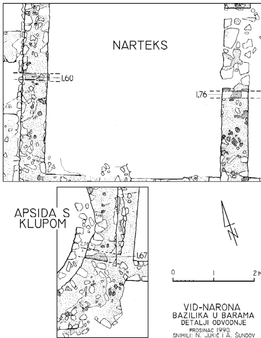
Sl. 37. Crkva u Erešovim barama: detalji odvodnog sustava (dokumentacija: Nada Jukić i Ante Šundov).
