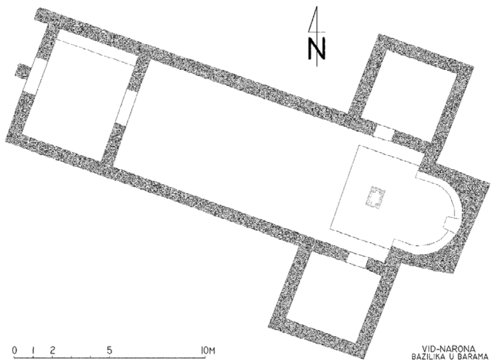
Sl. 45. Crkva u Erešovim barama: prijedlog rekonstrukcije (crtež: Branko Pender). Fig. 45. Église à Erešove bare: proposition de restitution (dessin: Branko Pender).
