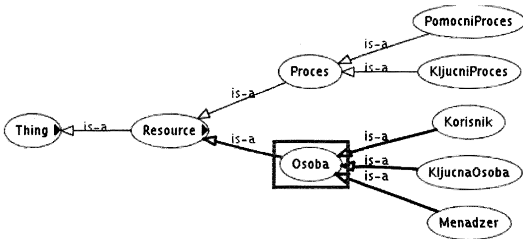
Slika 2. Djelomičan prikaz razvijene ontologije
