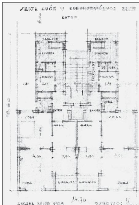
FIG. 2 5s AB PECINA, 6 KUKULJEVIĆEVA ST. ZG, 1939-40, PLAN
