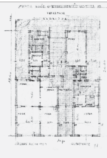
SL. 2. PETOETAŽNA UGRADENA NAJAMNA STAMBENA ZGRADA PECINA, KUKULJEVIĆEVA 6, ZG, 1939.-40., TLOCRT
