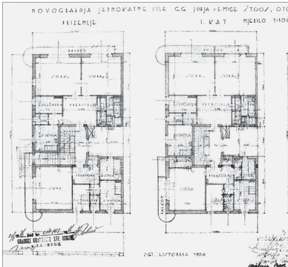
FIG. 3 5s V PICK&ŠTERK, O.&M.&ŠTOOS, 55 VOĆARSKA ST. ZG, 1936-37, PLANS
