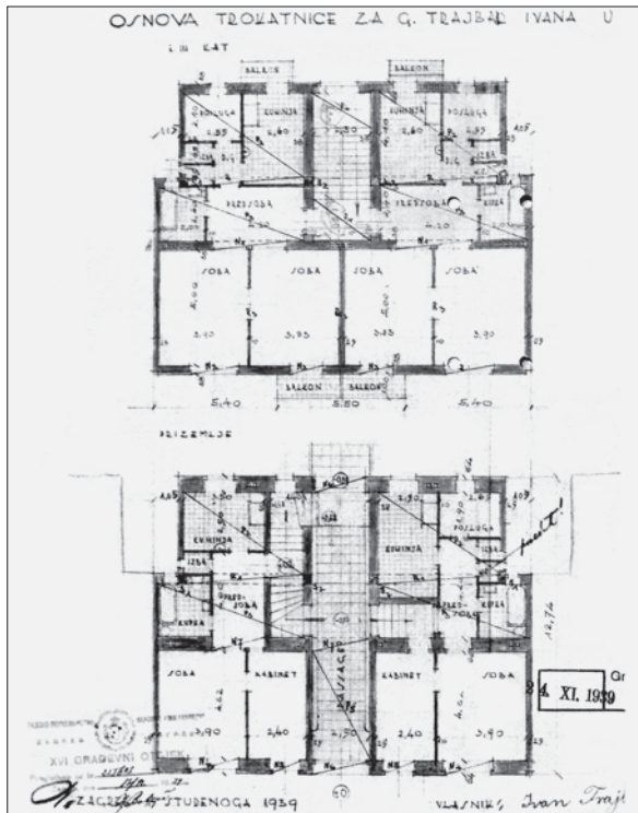
FIG. 4 5S AB TRAJBAR, 30 GRADA MAINZA ST. ZG, 1939-40, PLAN
