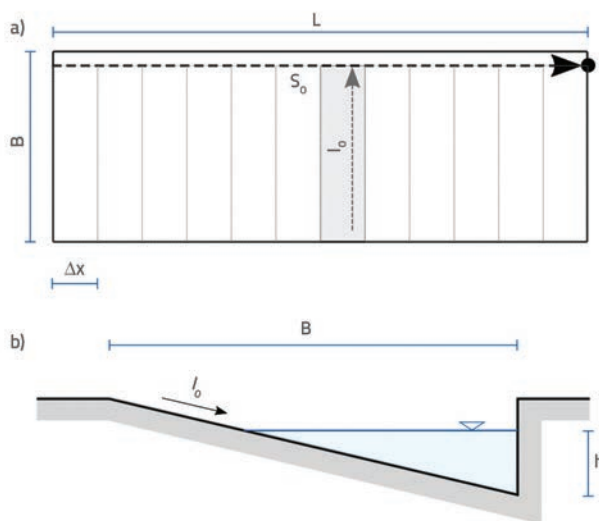
Slika 1. Shematski prikaz: a) tlocrtna površina izduženog pravokutnog sliva; b) karakterističnog poprečnog presjeka u smjeru otjecanja oborine
