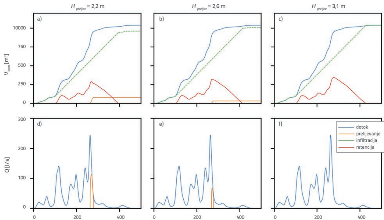
Slika 10. Promjene volumena vode u infiltracijskoj građevini tijekom ekstremne oborine iz kolovoza 1981. godine, dimenzioniranog na: a) ravnomjernu oborinu trajanja 1 h ( H_{\text{prelejev}} = 2,2 m), b) mjerodavnu oborinu trajanja 1 h ( H_{\text{prelejev}} = 2,6 m); c) mjerodavna oborina kritičnog trajanja ( H_{\text{prelejev}} = 3,1 m); d) do f) rezultirajuće promjene ulaznog i izlaznog protoka
