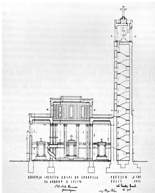
Slika 1. Presjek prve varijante projekta iz 1932. godine (Crnica, 1939: 467)
