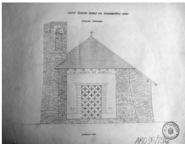
Slika 8. Perspektiva Kapele na Sljemeni (Arhiv HAZU)
