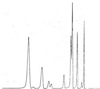
Primjer analize izomera C 4 - ugljikovodika
