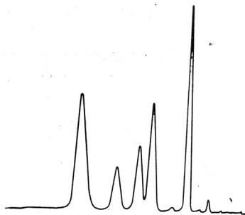
Zasićeni i nezasićeni metil esteri masnih kiselina C 12 do C 18
