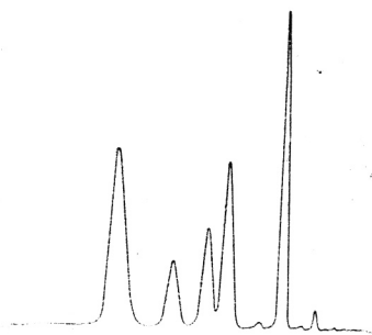
Zasićeni i nezasićeni metil esteri masnih kiselina C 12 do C 18
