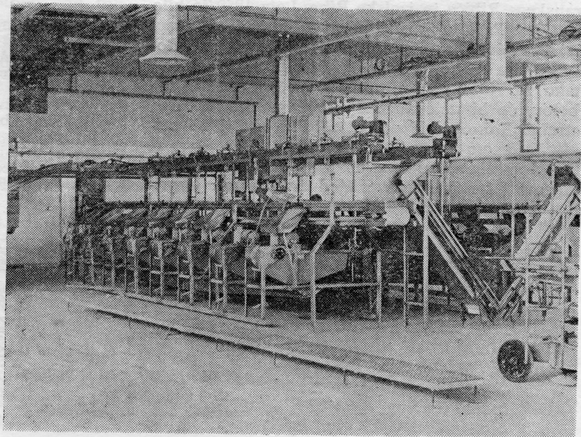
DO Droga Portorož, TOZD Delamaris — Izola, linija za rezanje in vlaganje rib v doze »Canarias«, 1985
