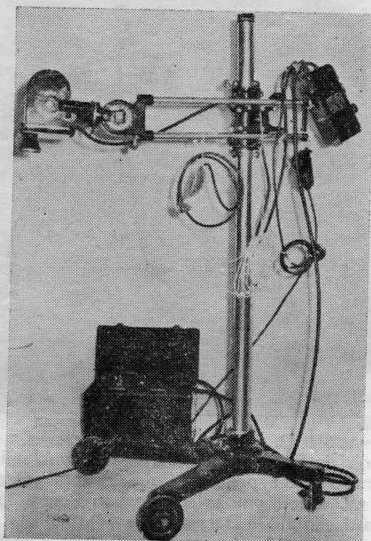
Sl: 10. Transportabilni Rentgen aparat
