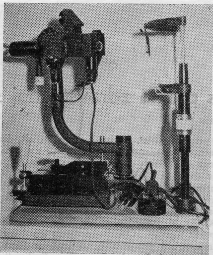
Sl: 3. Ophthalmometar po Javalu
