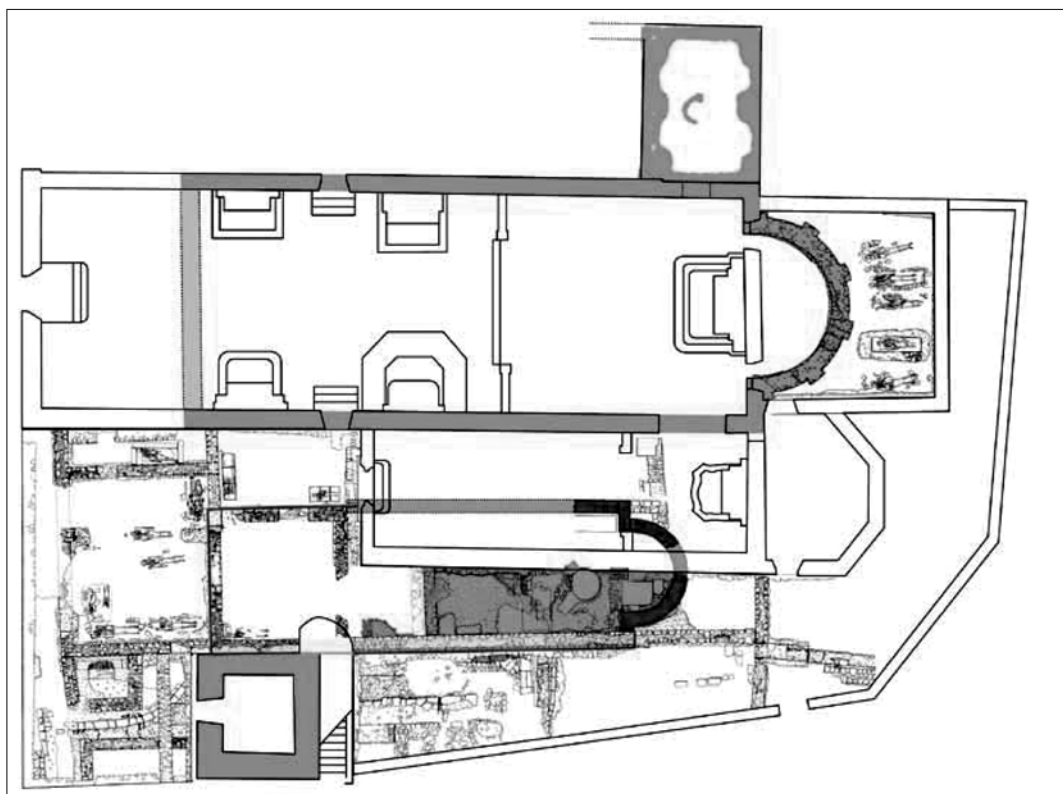
Slika 3. Episkopalni kompleks u Ninu, tlocrt, označeno žutom bojom: 5.-6. st.; označeno crvenom bojom: 7.-8. st.; označeno zelenom bojom: 12.-13. st. (izvor: M. KOLEGA 2014: 22)
