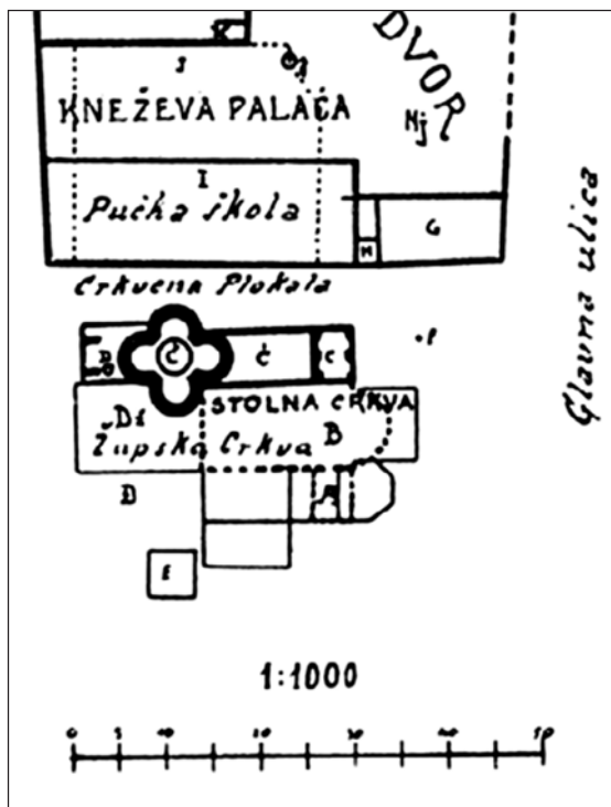
Slika 2. Episkopalni kompleks u Ninu, tlocrt (izvor: L. JELIĆ 1911: Tab. III., 3)
