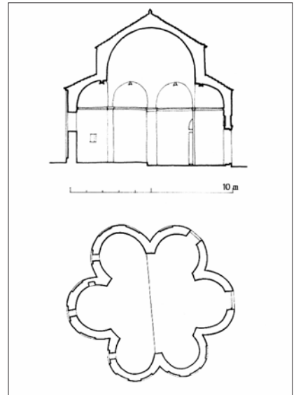
Slika 11. Presjek i tlocrt crkve Sv. Trojice u Splitu (izvor: P. VEŽIĆ 2012.)
