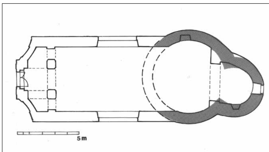
Slika 26. Orljavac, kapela sv. Roka, prikaz prve rotunde (Z. Horvat prema snimci D. Stepinca; A. Horvat, 1985)
