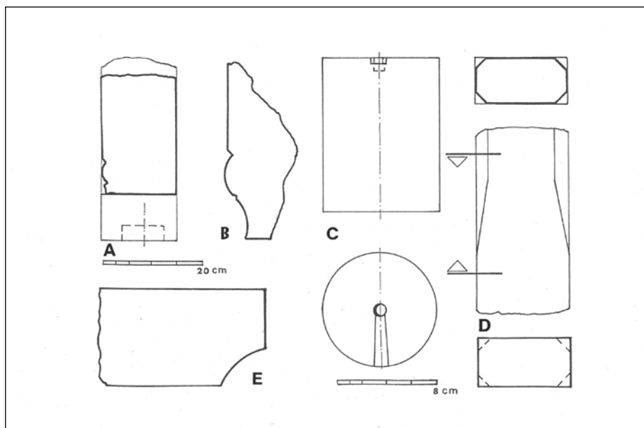
Slika 7. Lokalitet Njive – Ivandol, ulomci arhitektonske plastike (crtež: Z. Horvat)
