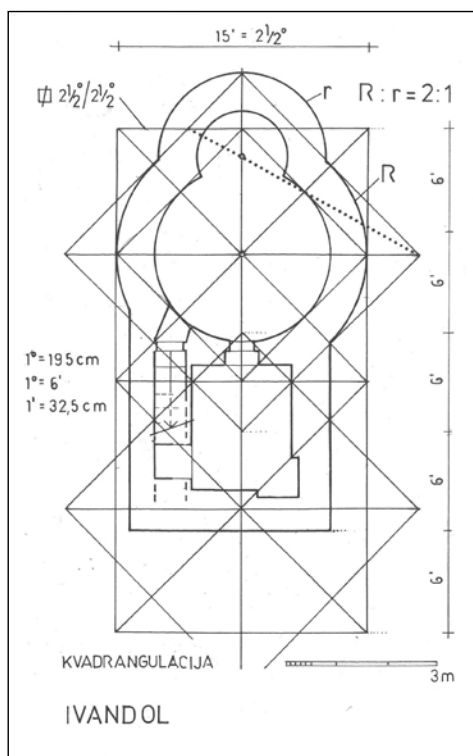
Slika 5. Lokalitet Njive – Ivandol, pokušaj kvadrangulacije rotunde (Z. Horvat)
