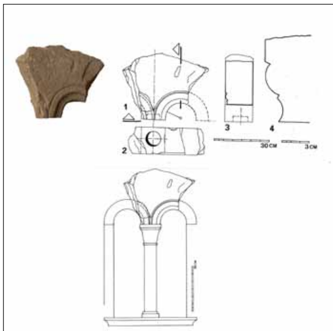
Slika 13. Lokalitet Njive – Ivandol, prikaz profilacija nekih kamenih ulomaka, nadvoj romaničke bifore, pogled i presjeci i pokušaj rekonstrukcije (crtež: Z. Horvat)
