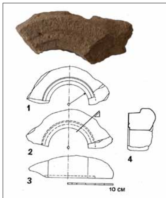
Slika 15. Lokalitet Njive – Ivandol, ulomak lučnog nadvoja, pogled i presjeci (crtež: Z. Horvat)
