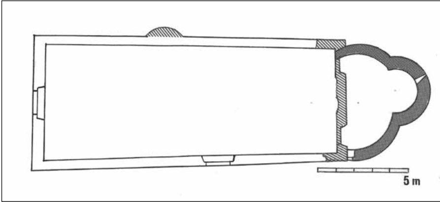
Slika 27. Mali Lž, kapela sv. Marije (crtež: S. Sekulić – Gozdanović 1978.)
