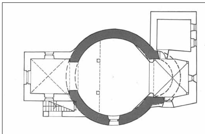
Slika 25. Otruševac kraj Samobora, kapela sv. Križa, tlocrt s prikazom prvotne apside (crtež: Z. Horvat prema snimci J. Živković 2007.)
