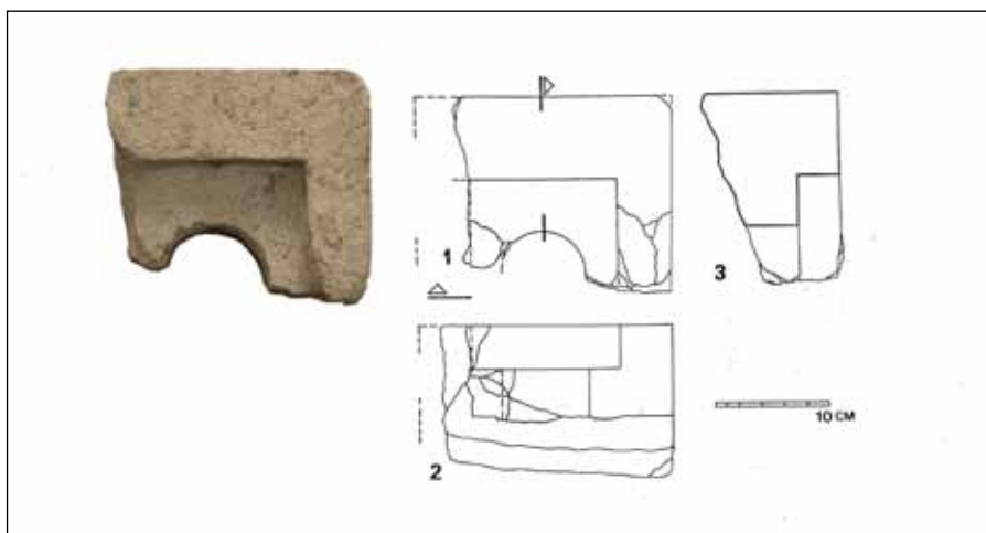
Slika 14. Lokalitet Njive – Ivandol, ulomak tranzene ili kružišta (?), pogled i presjeci (crtež Z. Horvat)
