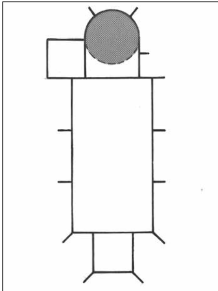
Slika 22. Samarica, župna crkva sv. Katarine, shematski prikaz uključivanja jedne rotunde u kasnogotičku, kasnije barokiziranu crkvu (crtež: Z. Horvat)
