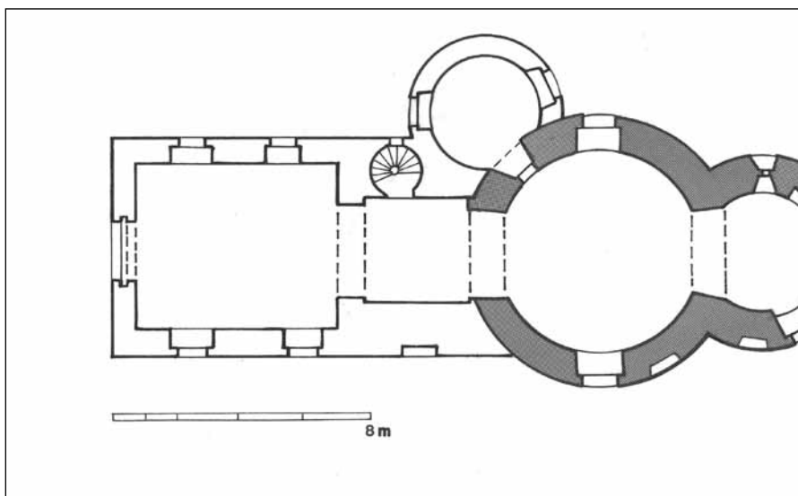
Slika 24. Gojilo – Kutina, kapelica Sv. Duha (crtež: Z. Horvat)
