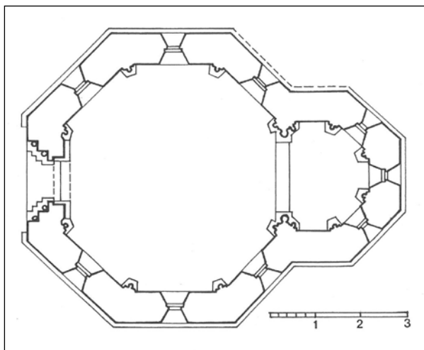
Slika 29. Medvedgrad, kapela sv. Filipa i Jakova, tlocrt (crtež: Z. Horvat prema Miletić – Valjato – Fabris, 1987.)
