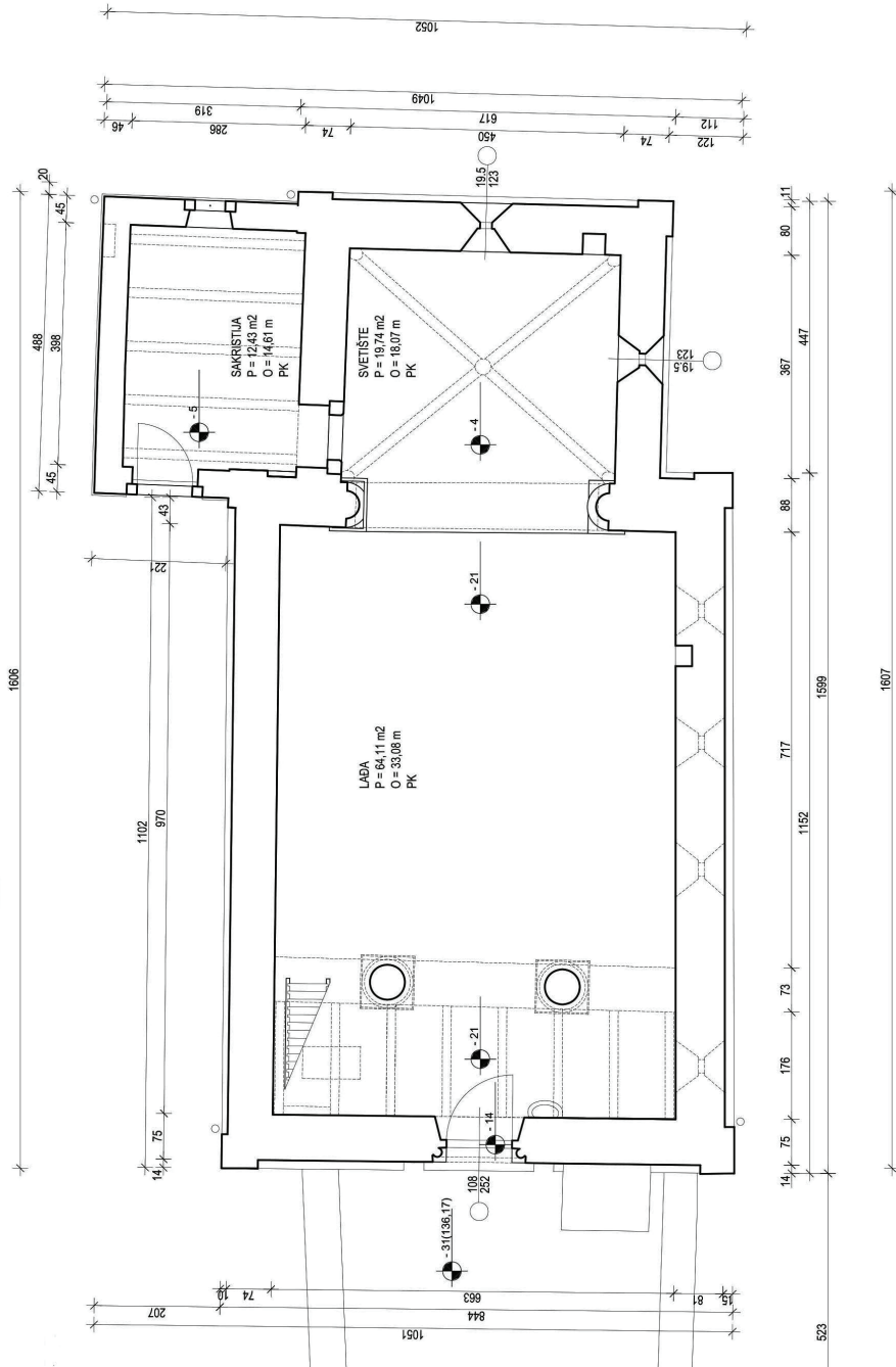
I. Novo Mjesto, kapela sv. Petra – tlocrt (crtača: Teodora Kućinać)
