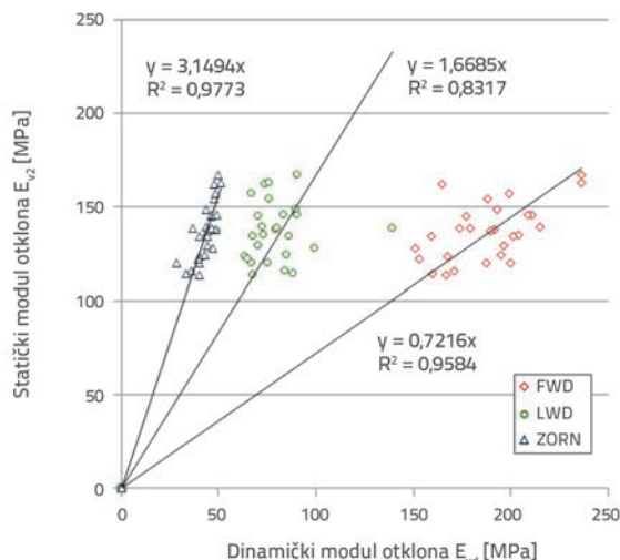
Slika 10. Regresijski modeli za izračun statičkog deformacijskog modula E_{vz} na osnovi vrijednosti deformacijskog modula E_{vd} dobivenog mjerenjem uređajima FWD, LWD i ZORN
