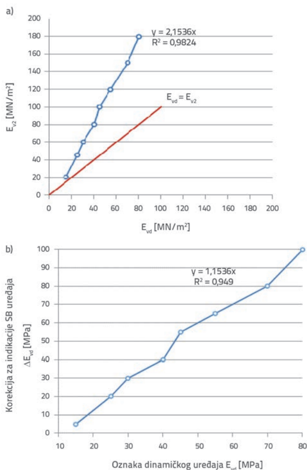
Slika 3. Linearna ovisnost statičkog deformacijskog modula E_{v2} o dinamičkom deformacijskom modulu E_{vd} : a) apsolutne vrijednosti; b) dodane korekcijske vrijednosti
