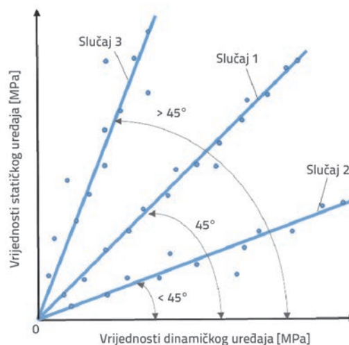
Slika 2. Korelacijski modeli očitavanja statičkih i dinamičkih uređaja: (Slučaj 1: oba očitavanja su približno ista, Slučaj 2: očitavanja statičkog uređaja su niža od očitavanja dinamičkog uređaja, Slučaj 3: očitavanja statičkog uređaja imaju veće vrijednosti od očitavanja dinamičkog uređaja)
