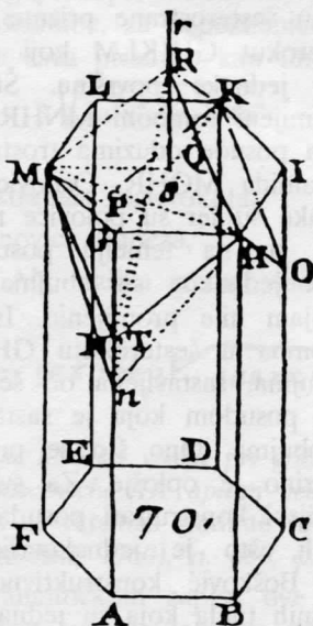
Sl. 3. Oplošje stanice pčelinjega saća: ploha najmanje površine među prizmatičnim plohama koje omeđuju unaprijed određeni obujam. Boscovich, "De apium cellulis", u: Benedictus Stay, Philosophiae recentioris ... versibus traditae libri X, Tomus II. (Romae: Pagliarini, 1760), Tab. III., fig. 70.
