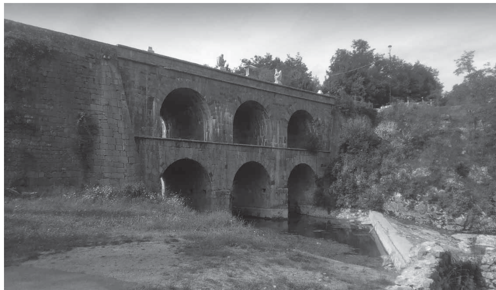
Slika 6: Tounjski most (na trasi Jozefinske ceste) u općini Tounj
